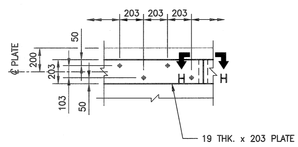
SECTION G-G SCALE: 1:20
