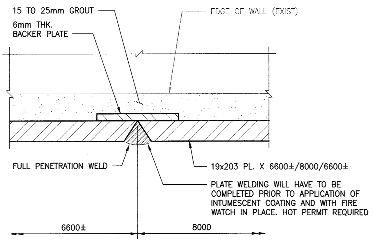
SECTION H-H SCALE: 1:2
