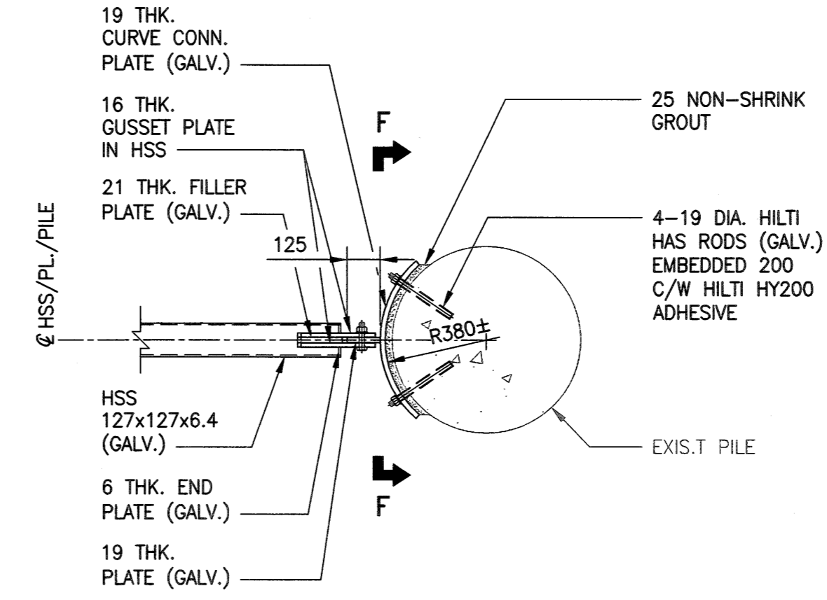
SECTION E-E SCALE: 1:20
