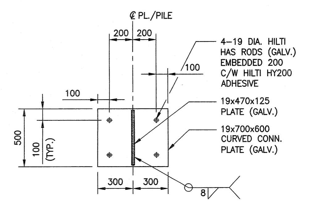
SECTION F-F SCALE: 1:20
