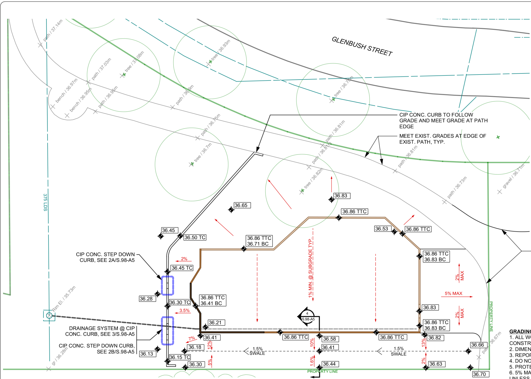
1 GRADING PLAN S.98-A4 Scale: 1:200
