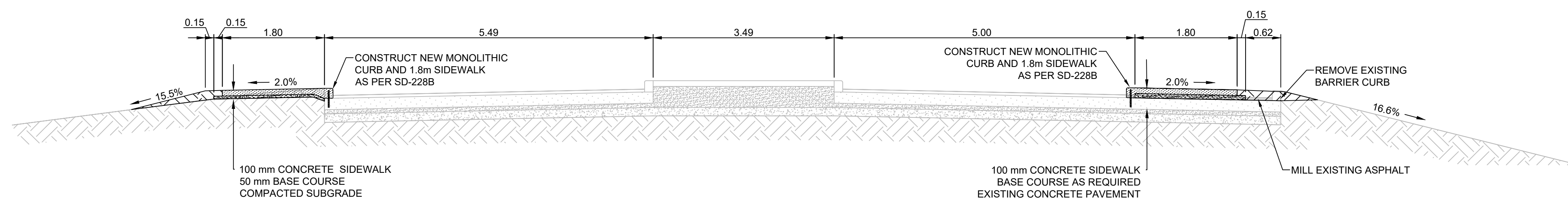
A WELLINGTON CRES CROSS SECTION N.T.S.
