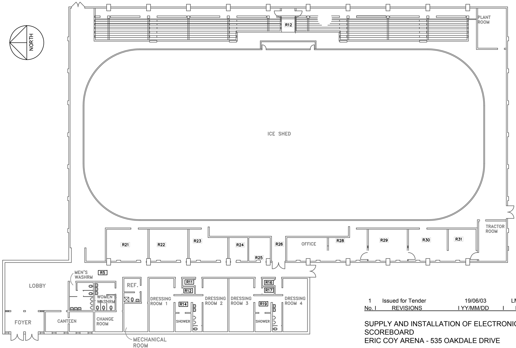
FLOOR PLAN LAYOUT SCALE: N.T.S.
