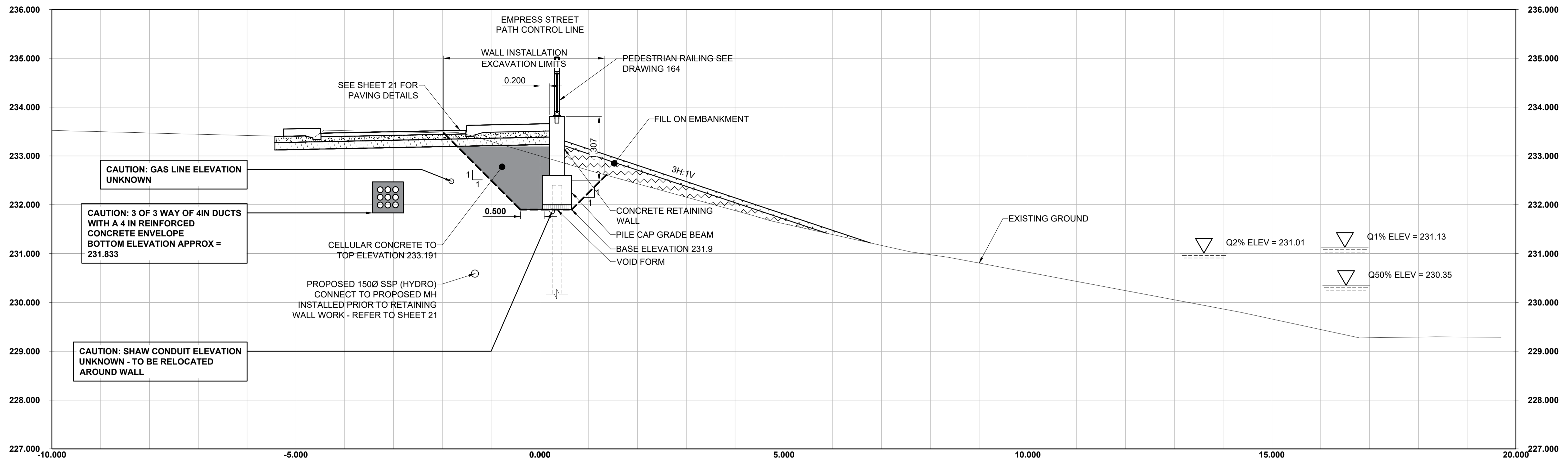
SECTION STA 1+673 0 SCALE: 1:50 H 5m 0 SCALE 1:50 V 5m
