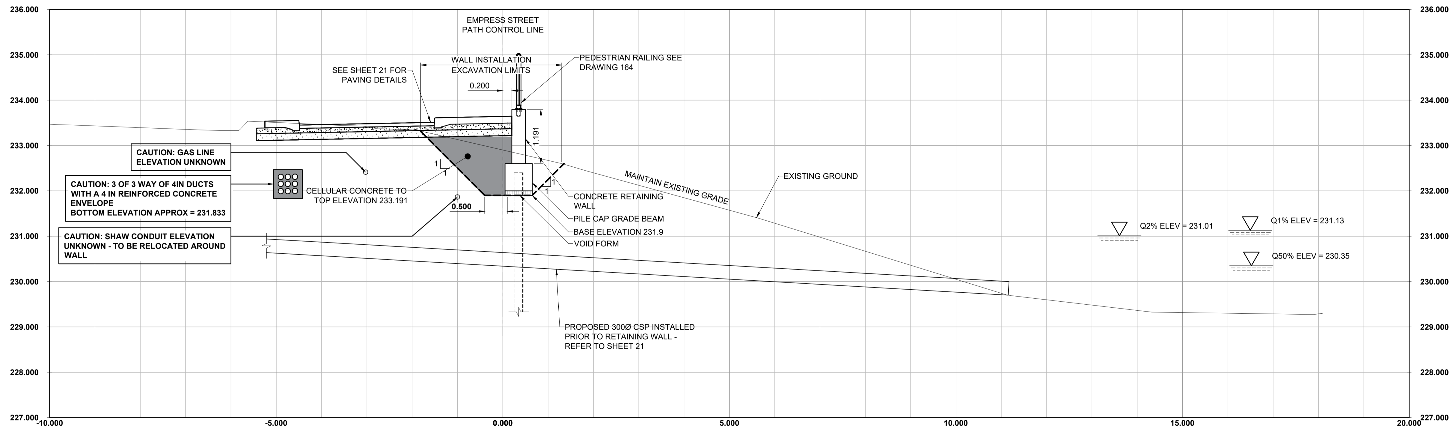
SECTION STA 1+682.15 0 SCALE: 1:50 H 5m 0 SCALE 1:50 V 5m
