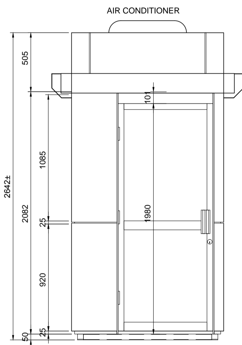
3 ELEVATION E-01 1:20
