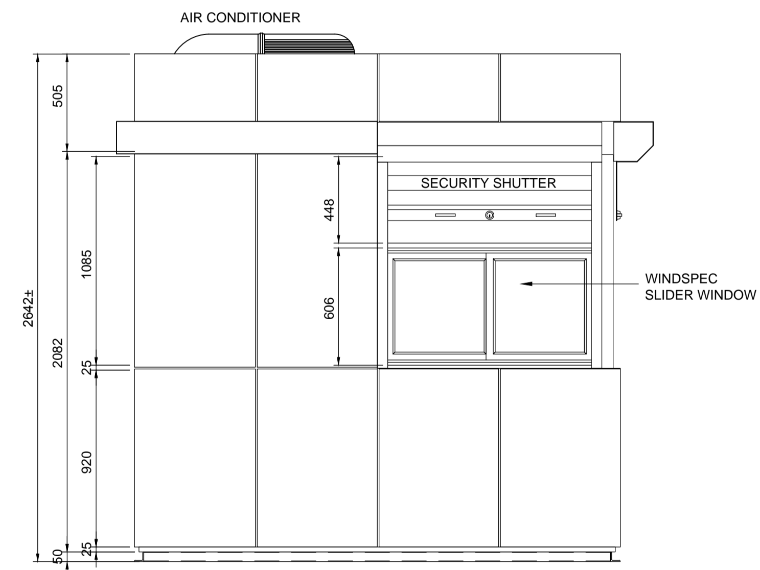
4 ELEVATION E-01 1:20
