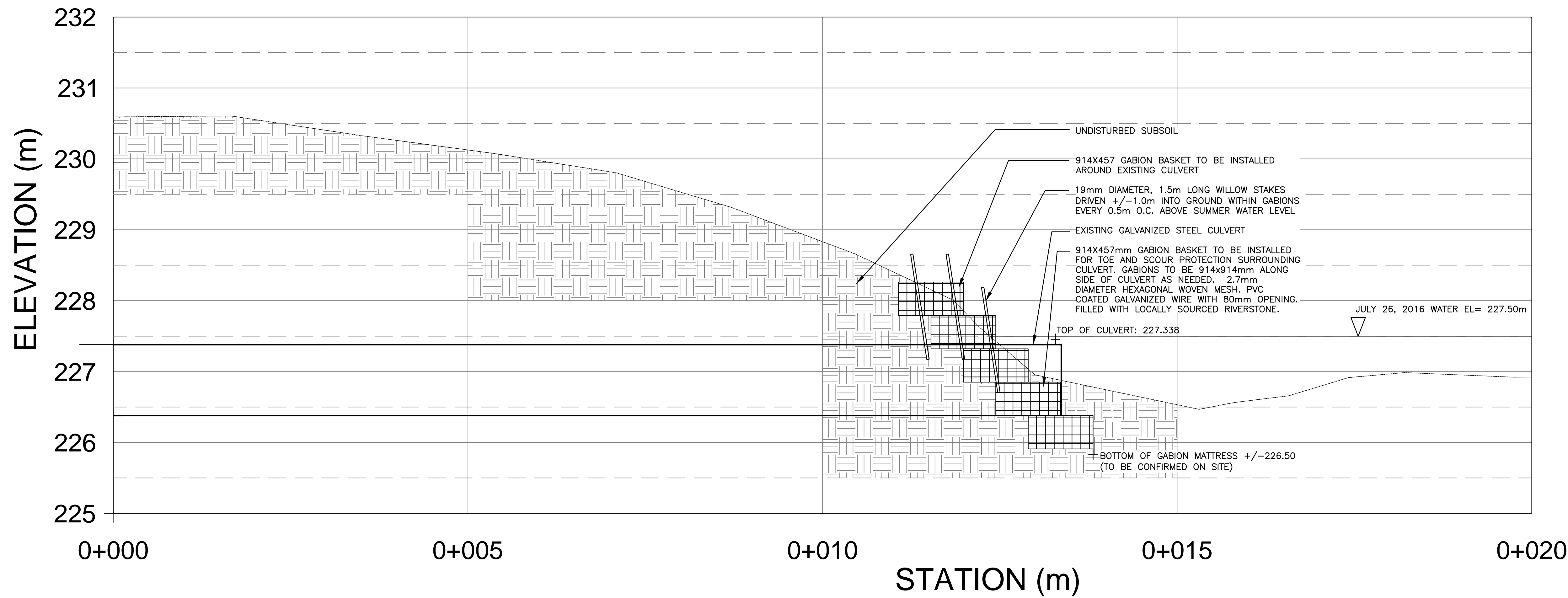
5 OUTFALL #2: SECTION B-B L3.2 N.T.S.
