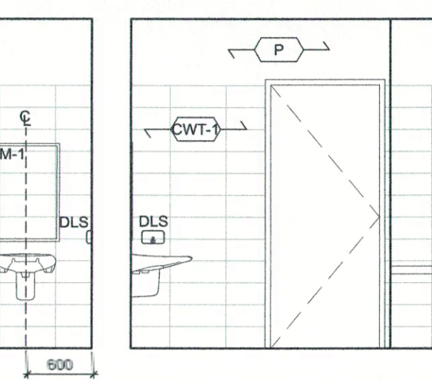
8 UTR 116 A-402 1:50
