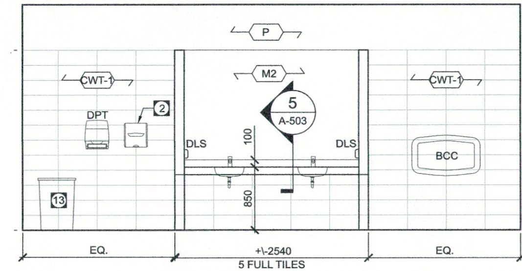
1 MEN W/C 115 A-402 1:50
