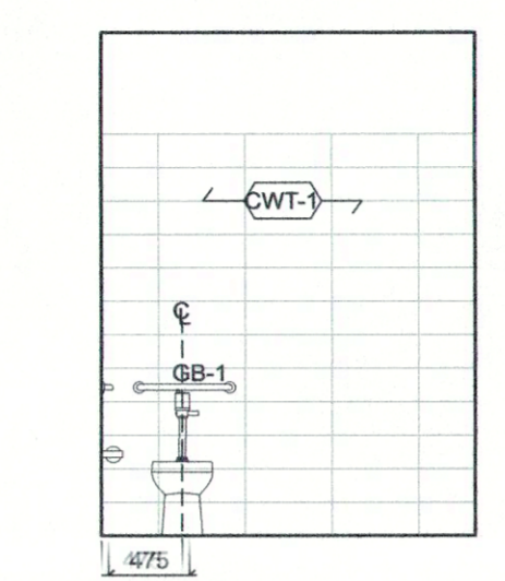
4 MEN W/C 115 A-402 1:50
