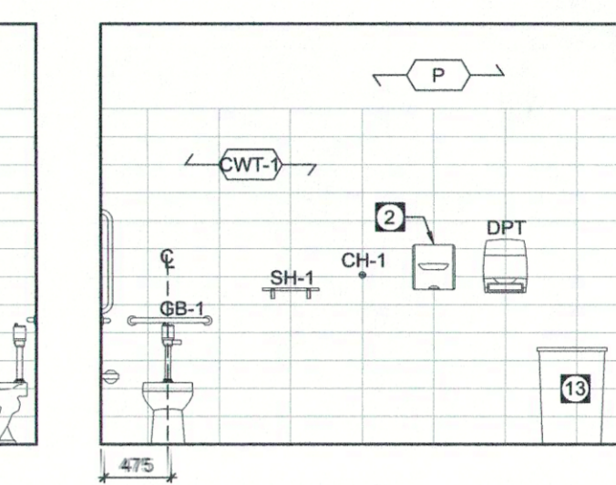
7 UTR 116 A-402 1:50
