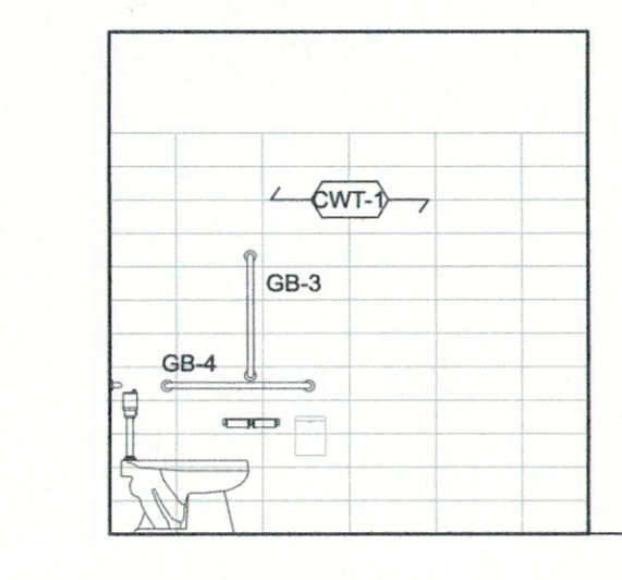
5 MEN W/C 115 A-402 1:50
