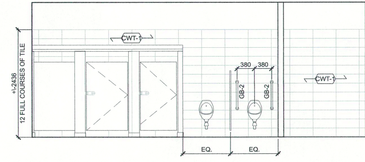
2 MEN W/C 115 A-402 1:50
