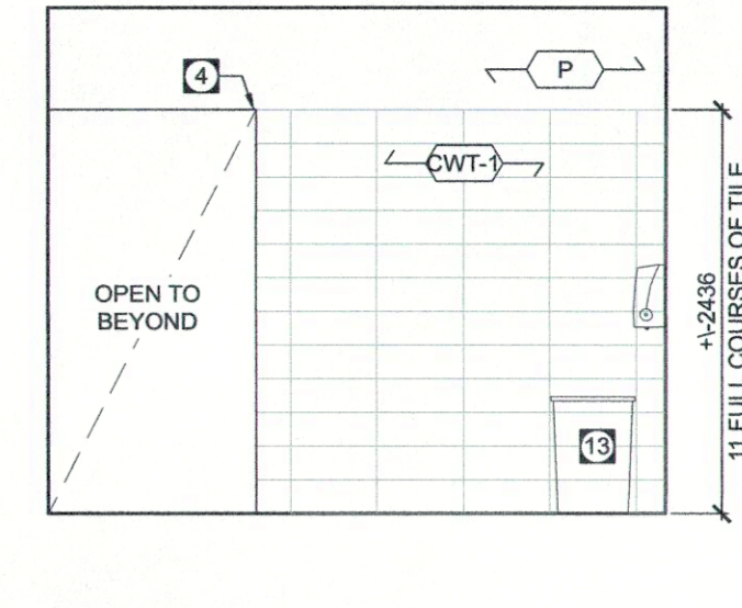
3 MEN W/C 115 A-402 1:50
