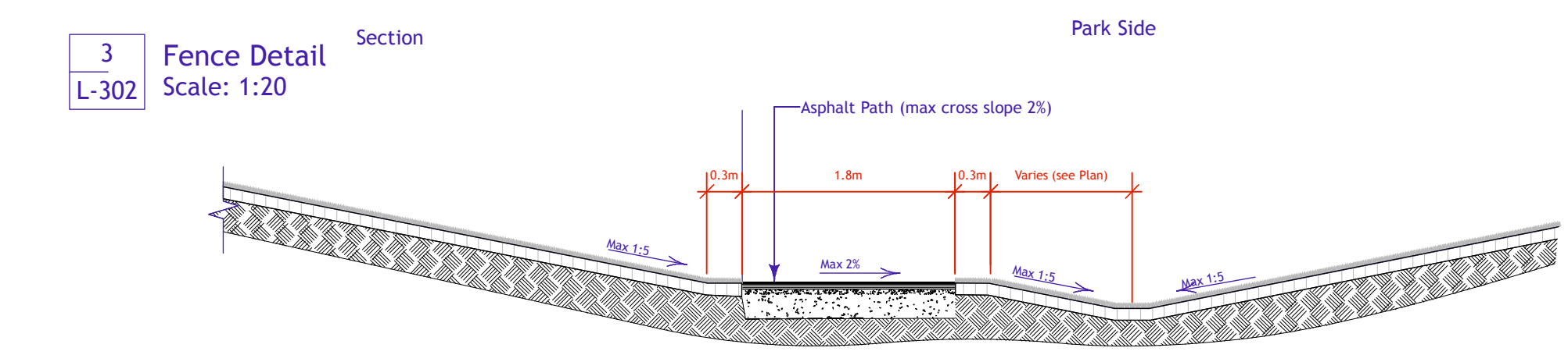
3 Fence Detail L-302 Scale: 1:20
