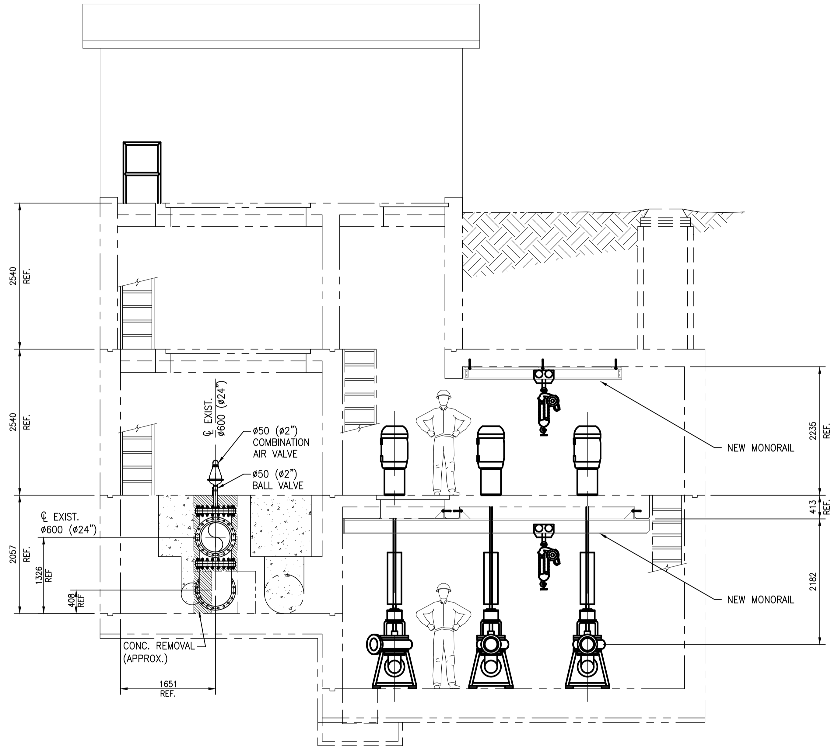
A SECTION SCALE: 1 : 40
