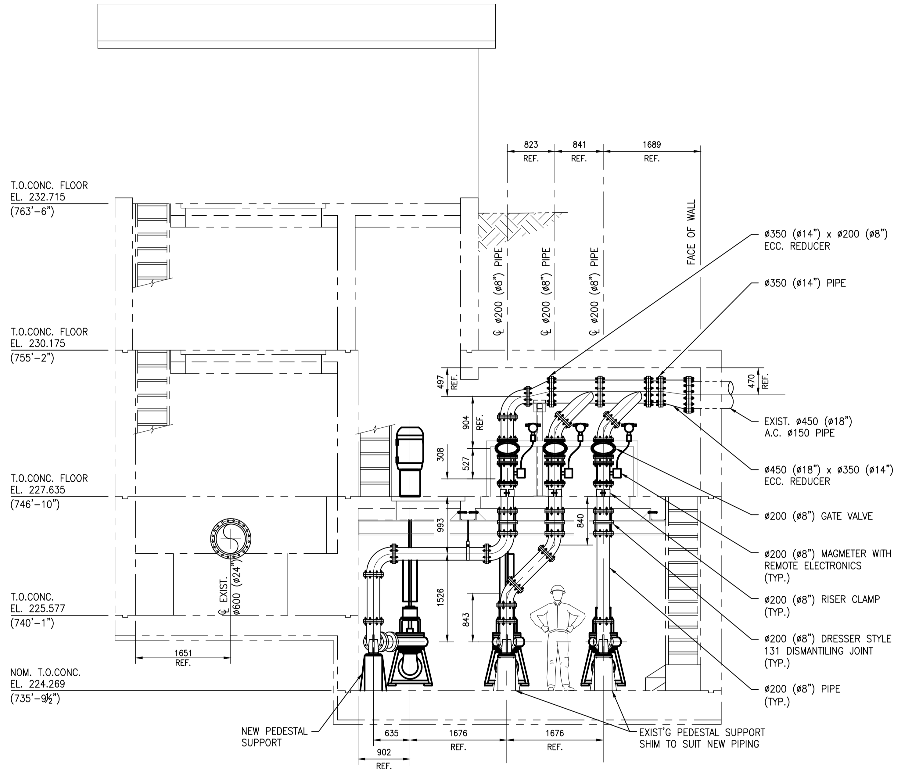
B SECTION SCALE: 1 : 40
