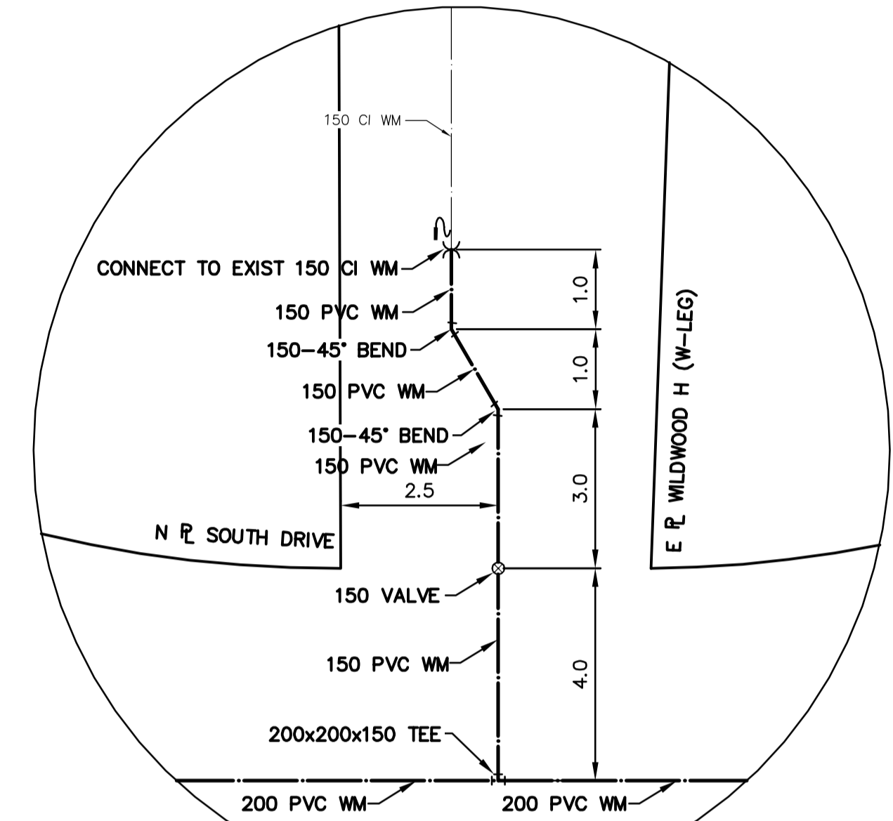
DETAIL "B" SCALE: NTS
