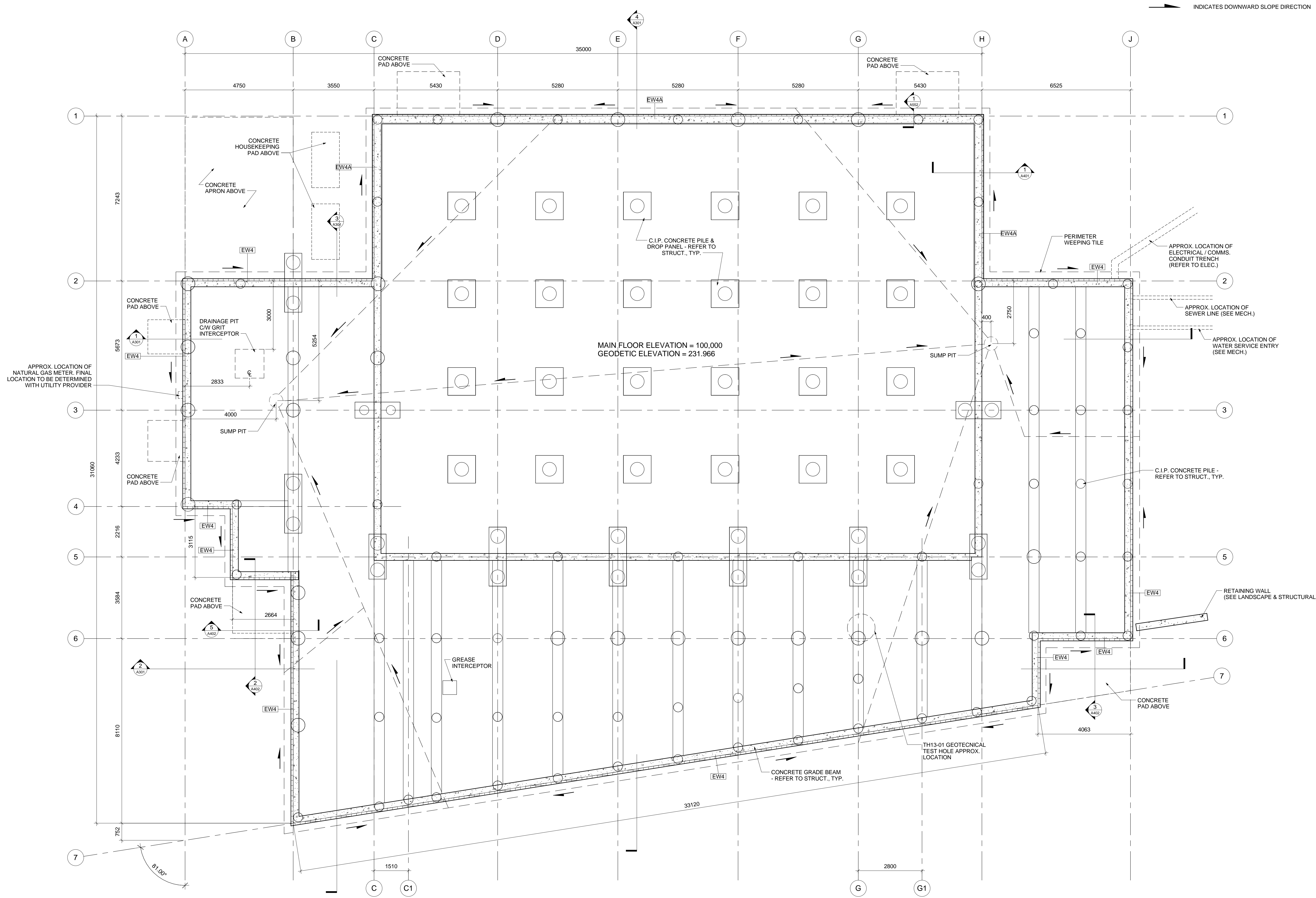
1 FOUNDATION PLAN 1 : 75
