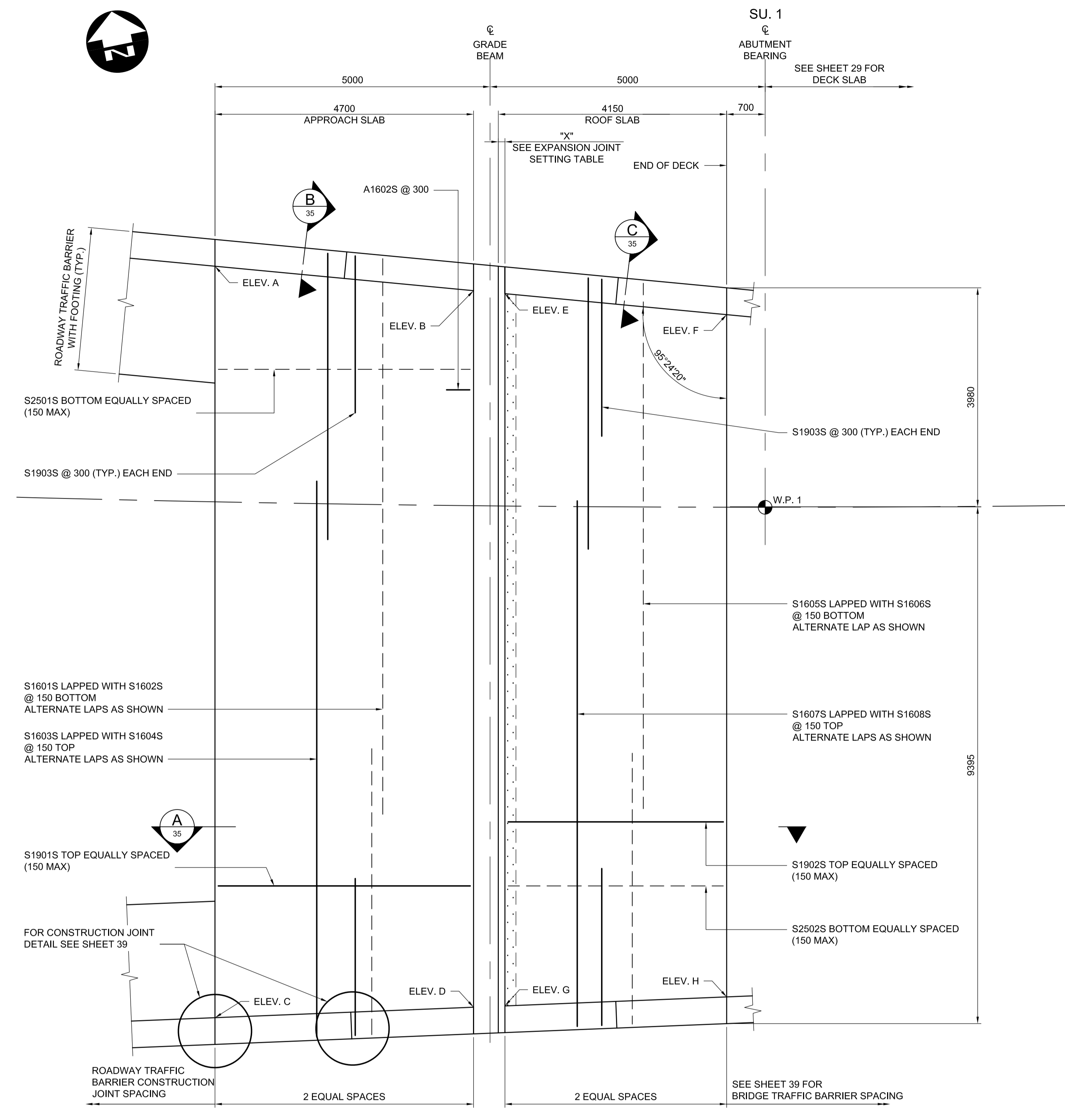
PLAN 1:50
