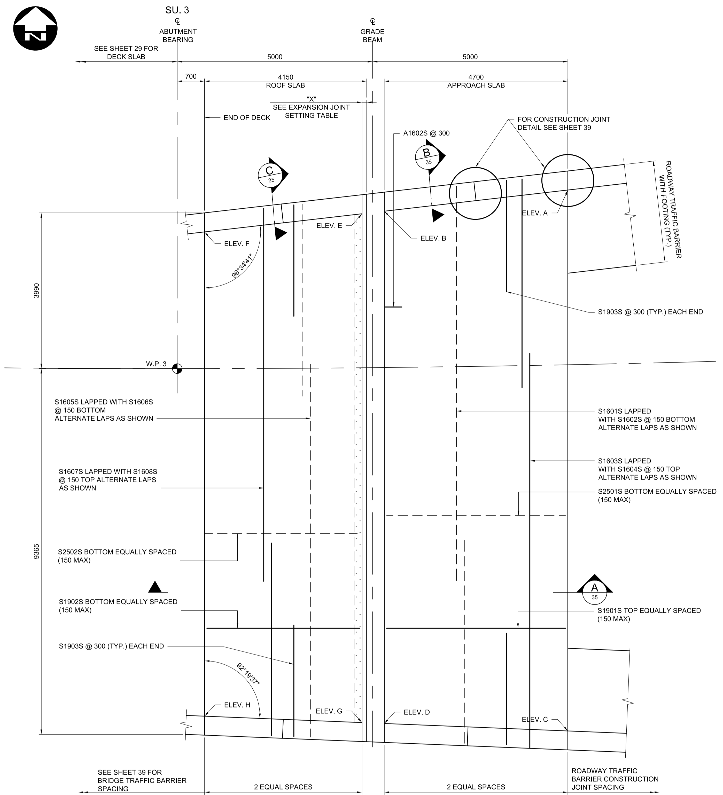
PLAN 1:50
