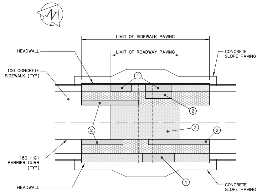
C-368 DESJARDINS DRIVE CULVERT N.T.S.
