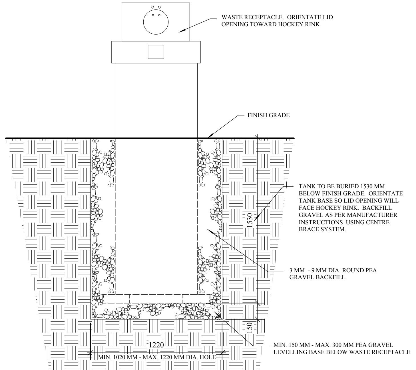
1 WASTE RECPTACLE SECTION L-4 Scale: 1:20
