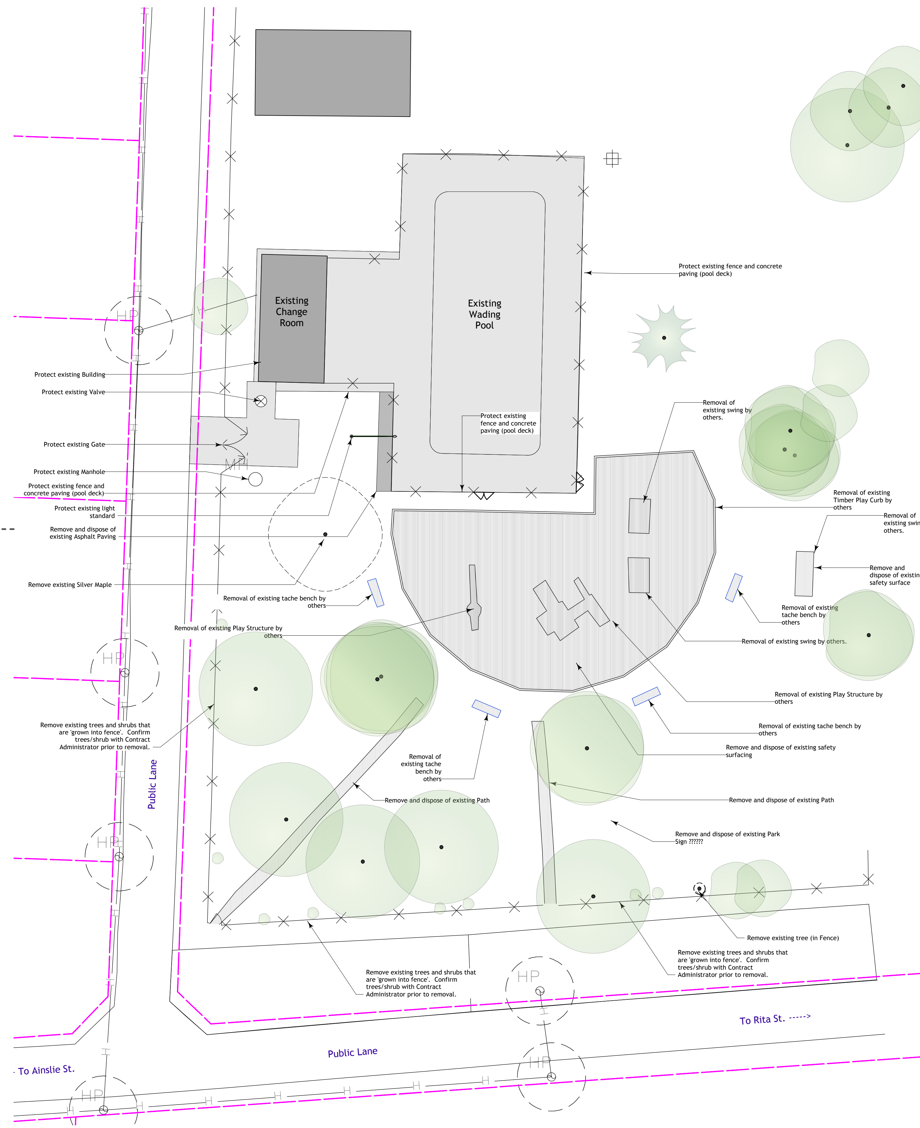
1 Site Demolition Plan L-4 Scale: 1:200
