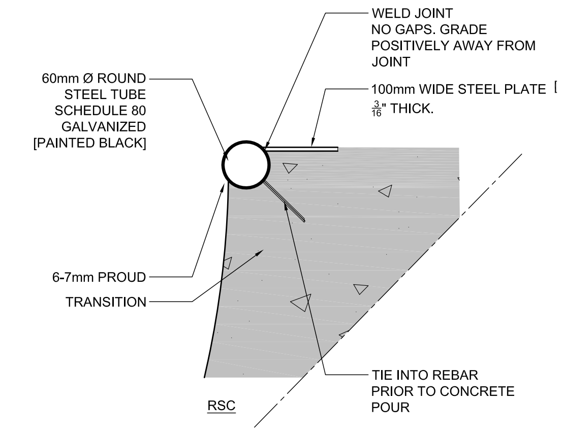
3 COPING PLACEMENT L9 SCALE - 1 : 5
