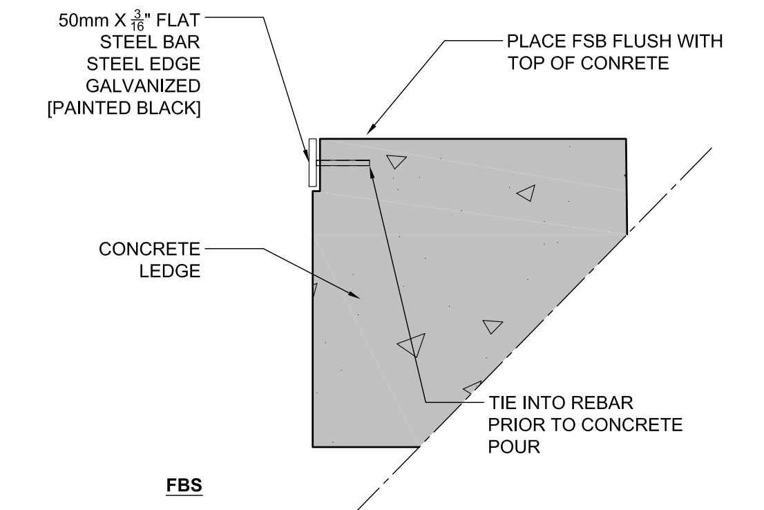
4 FLAT BAR STEEL EDGE L9 SCALE - 1 : 5
