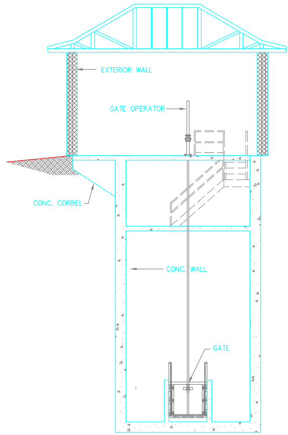
LONGITUDINAL SECTION
