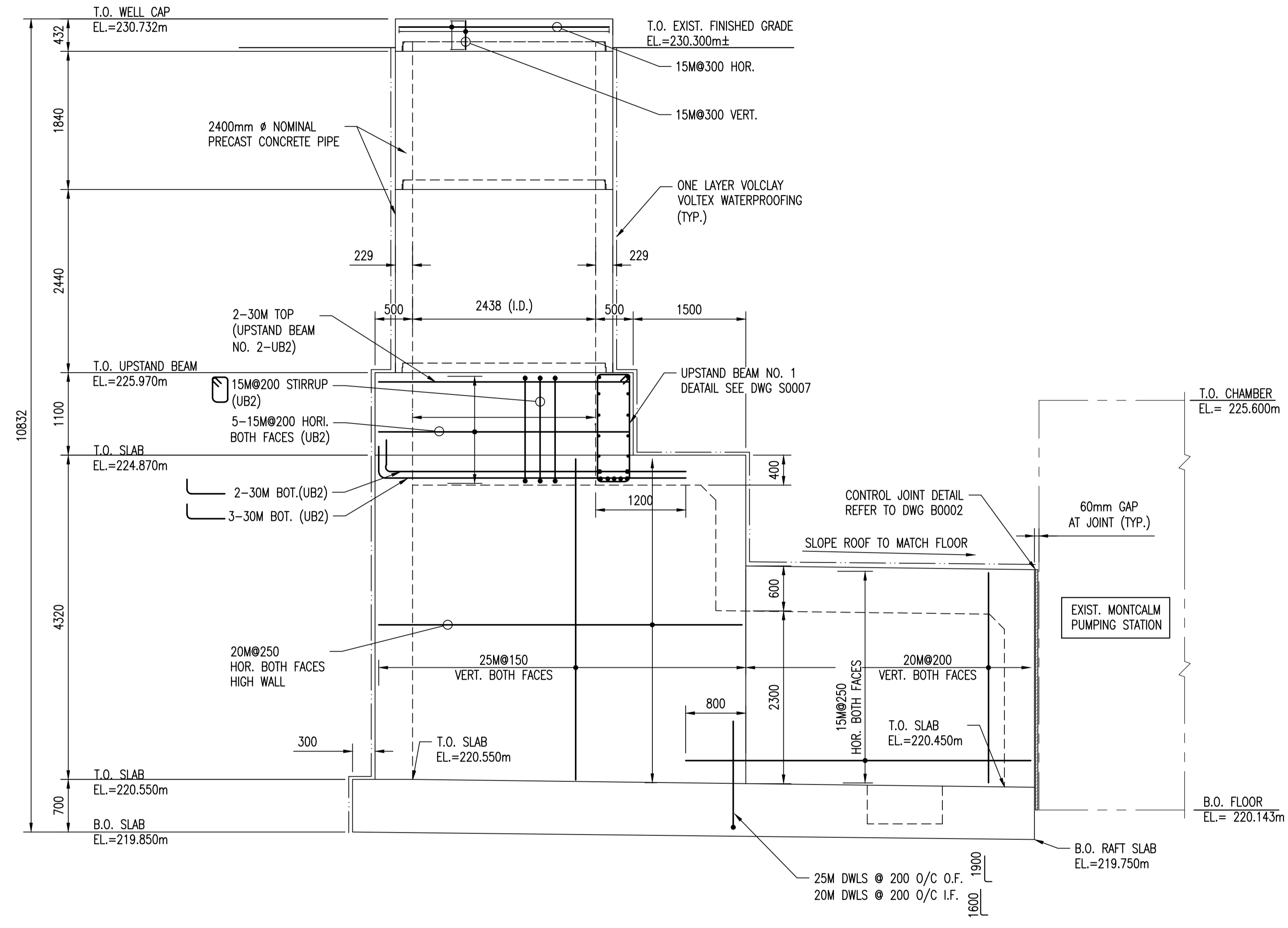
1 1 S0002 S0003 ELEVATION SCALE: 1 : 40
