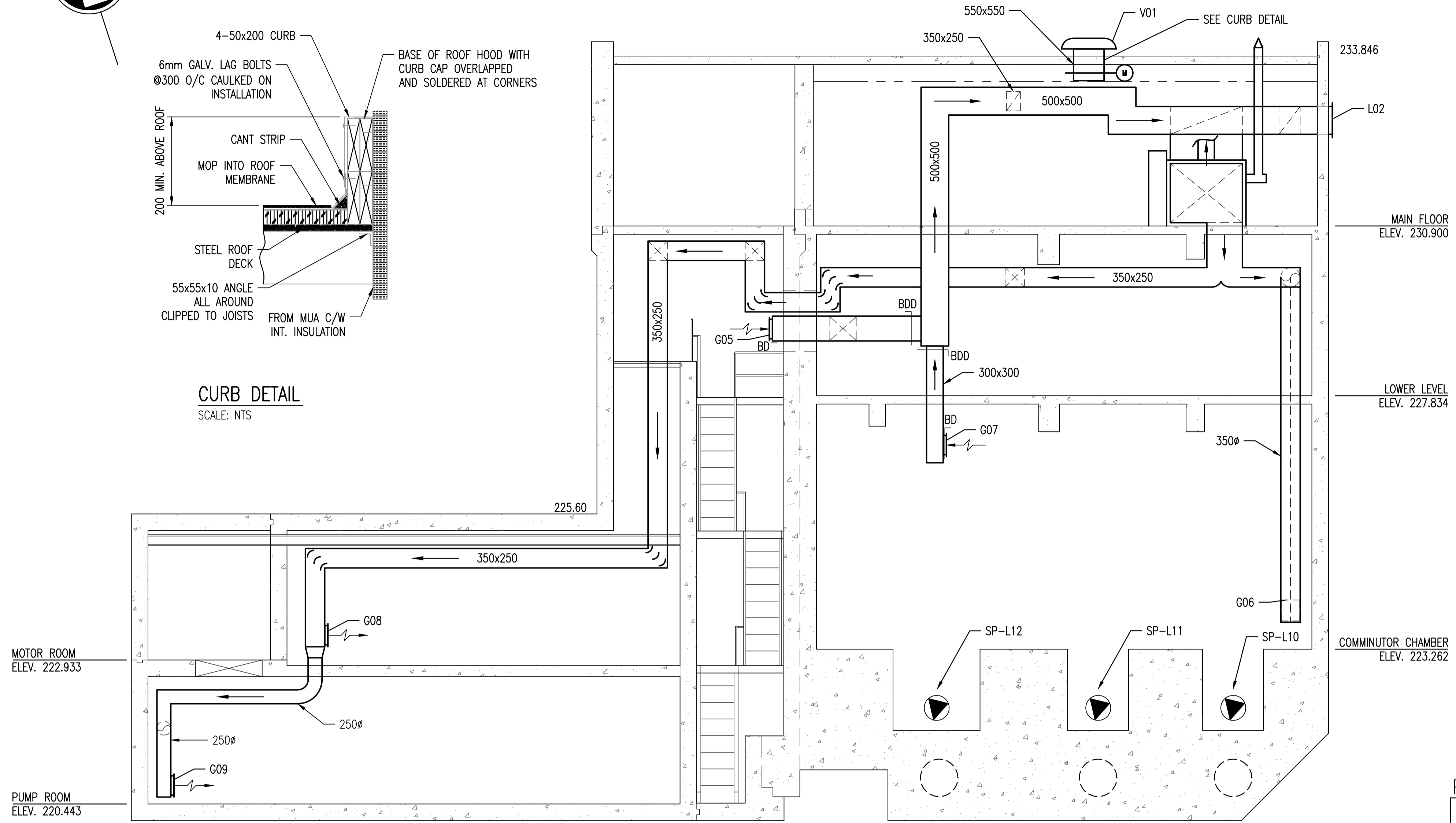
SECTION A SCALE: 1 : 50
