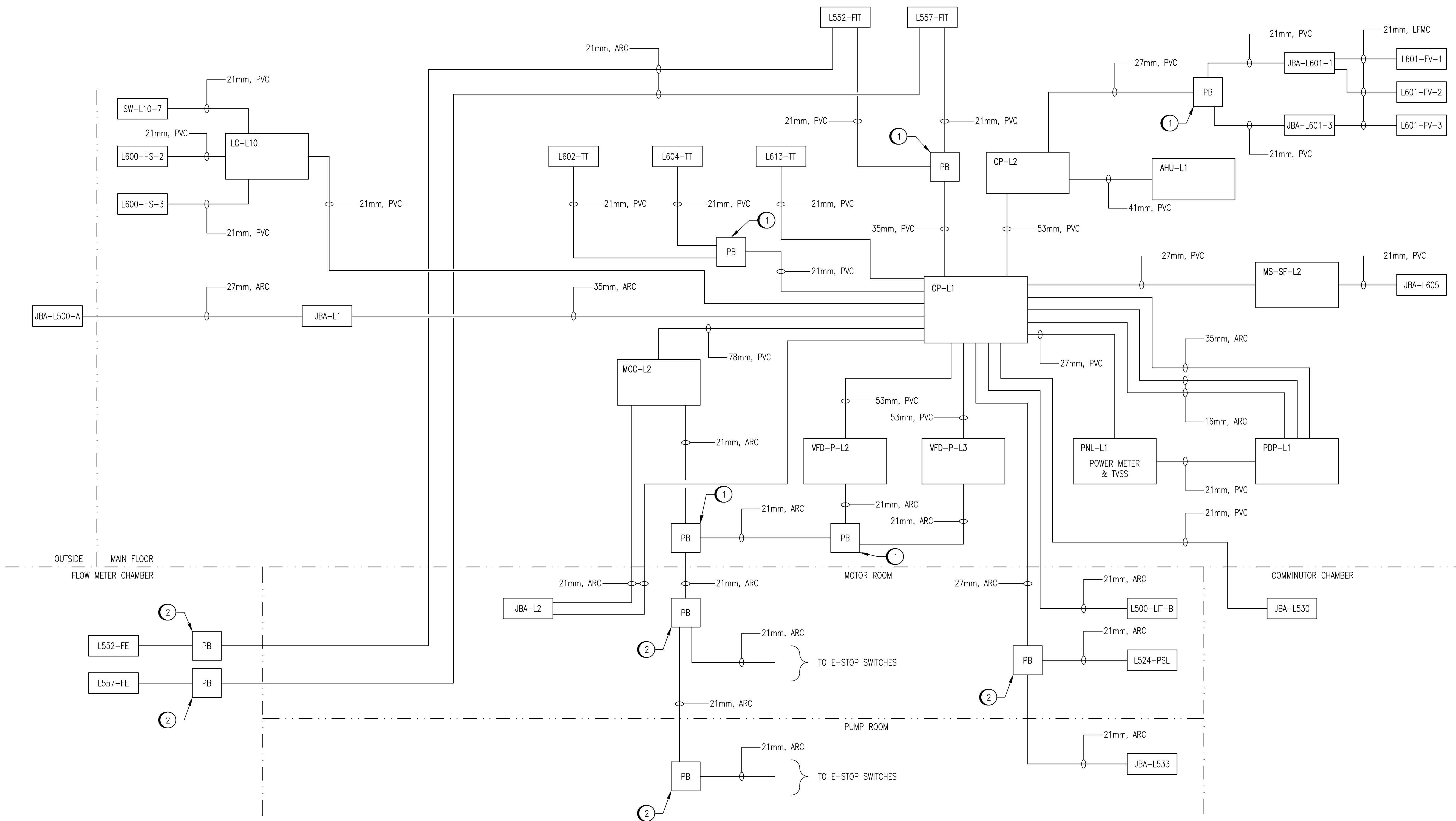
AUTOMATION CONDUIT RISER DIAGRAM SCALE: NTS
