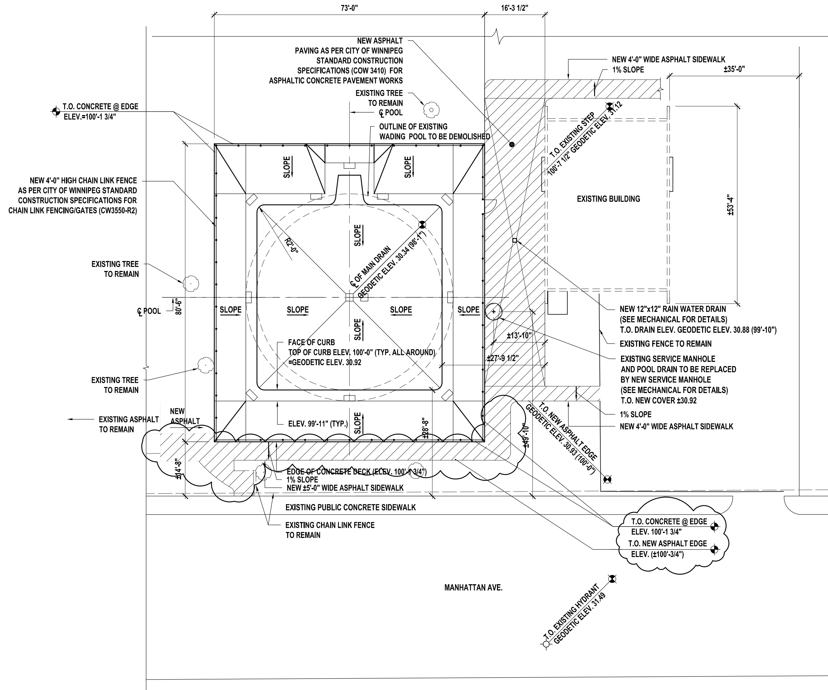
SITE PLAN Scale = 1/16" = 1'-0" 1 A1 | A1
