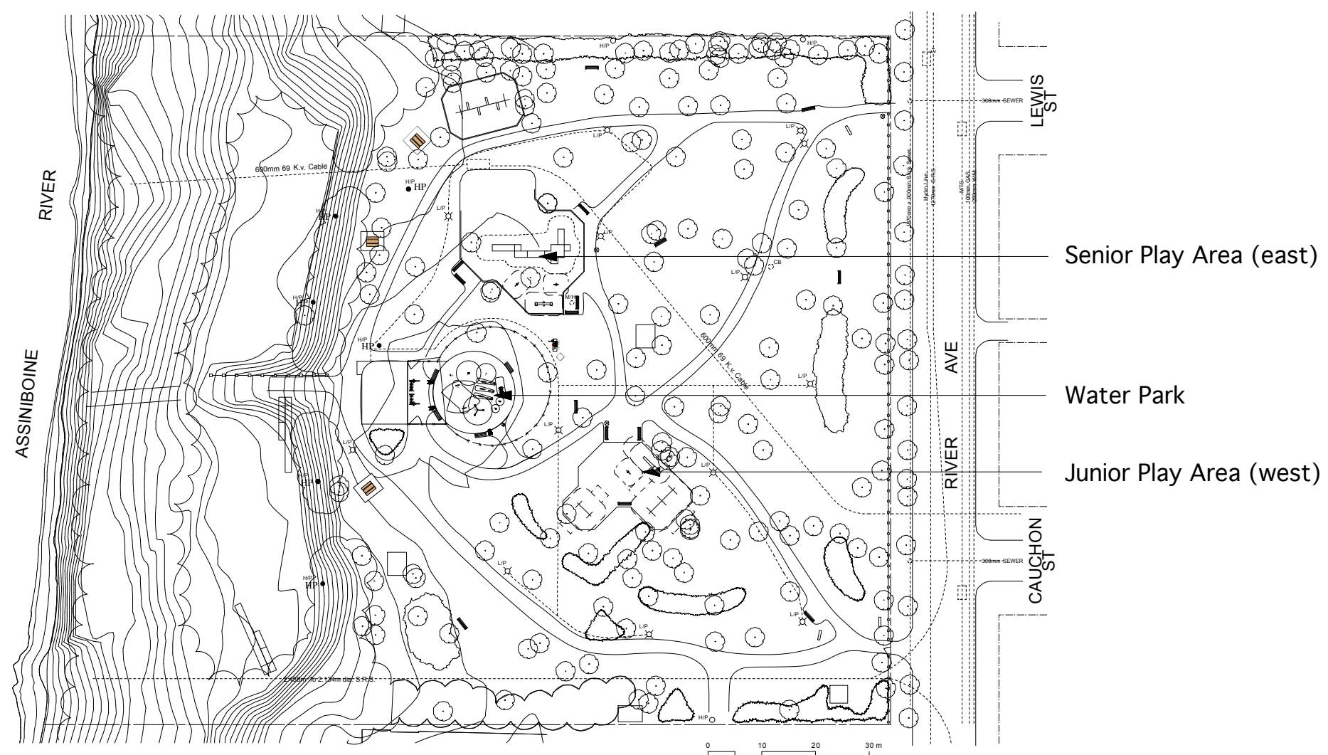
1 L1 CONTEXT PLAN Scale: 1:1000
