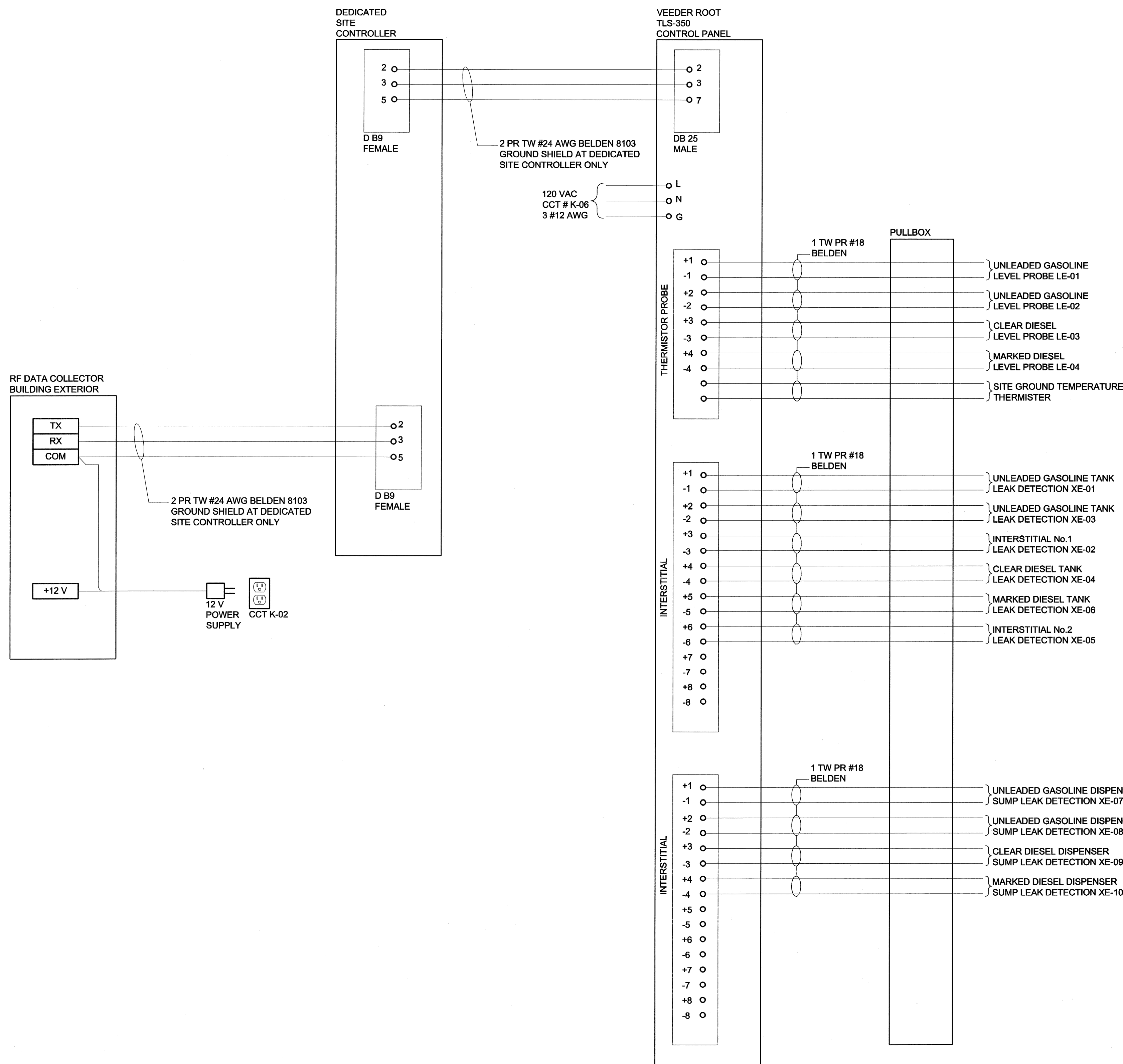
DEDICATED SITE CONTROLLER SCALE: N.T.S.
