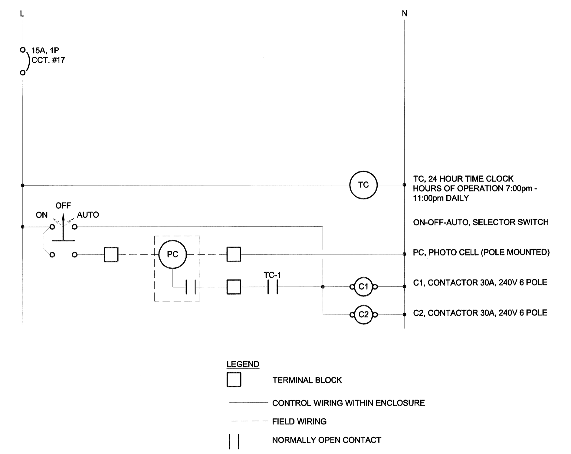
CONTROL SCHEMATIC SCALE: N.T.S.
