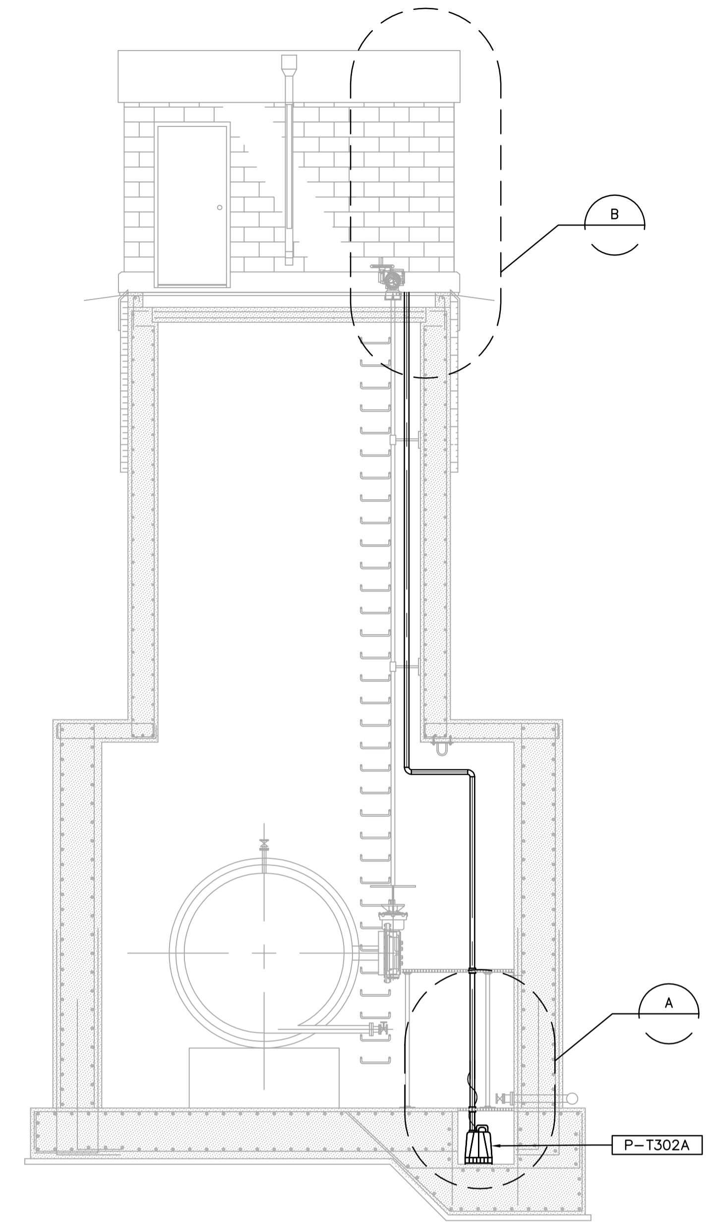
3 SECTION WY-H0403 1:50
