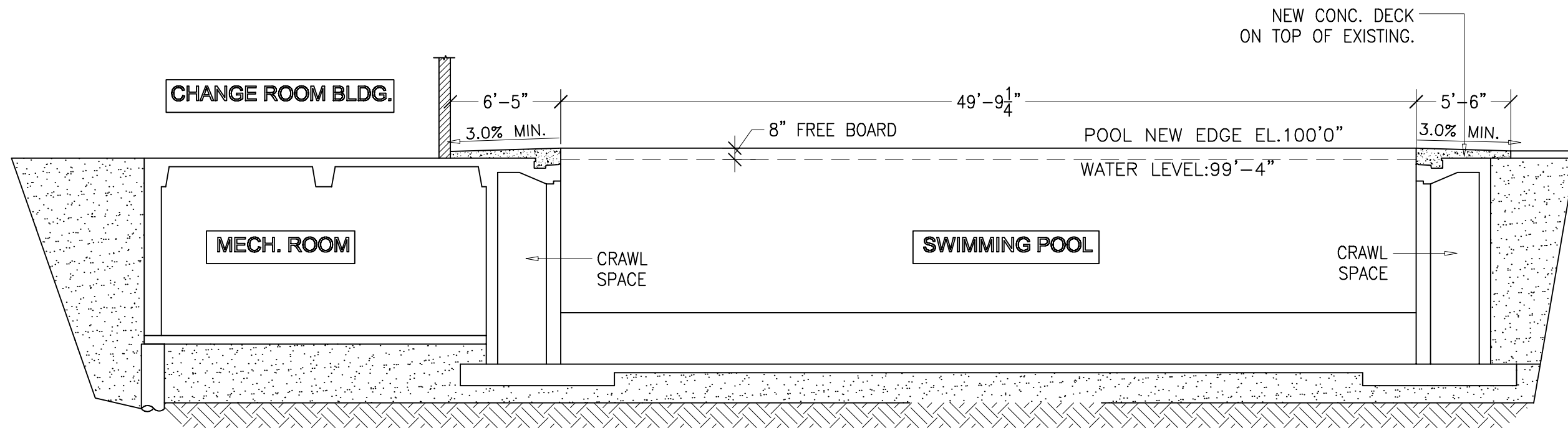
2 POOL SECTION-2 A2 | A3
