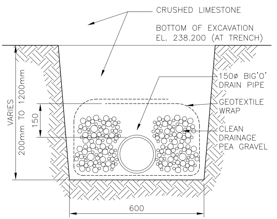
1 SECTION - TRENCH SCALE: 1:10
