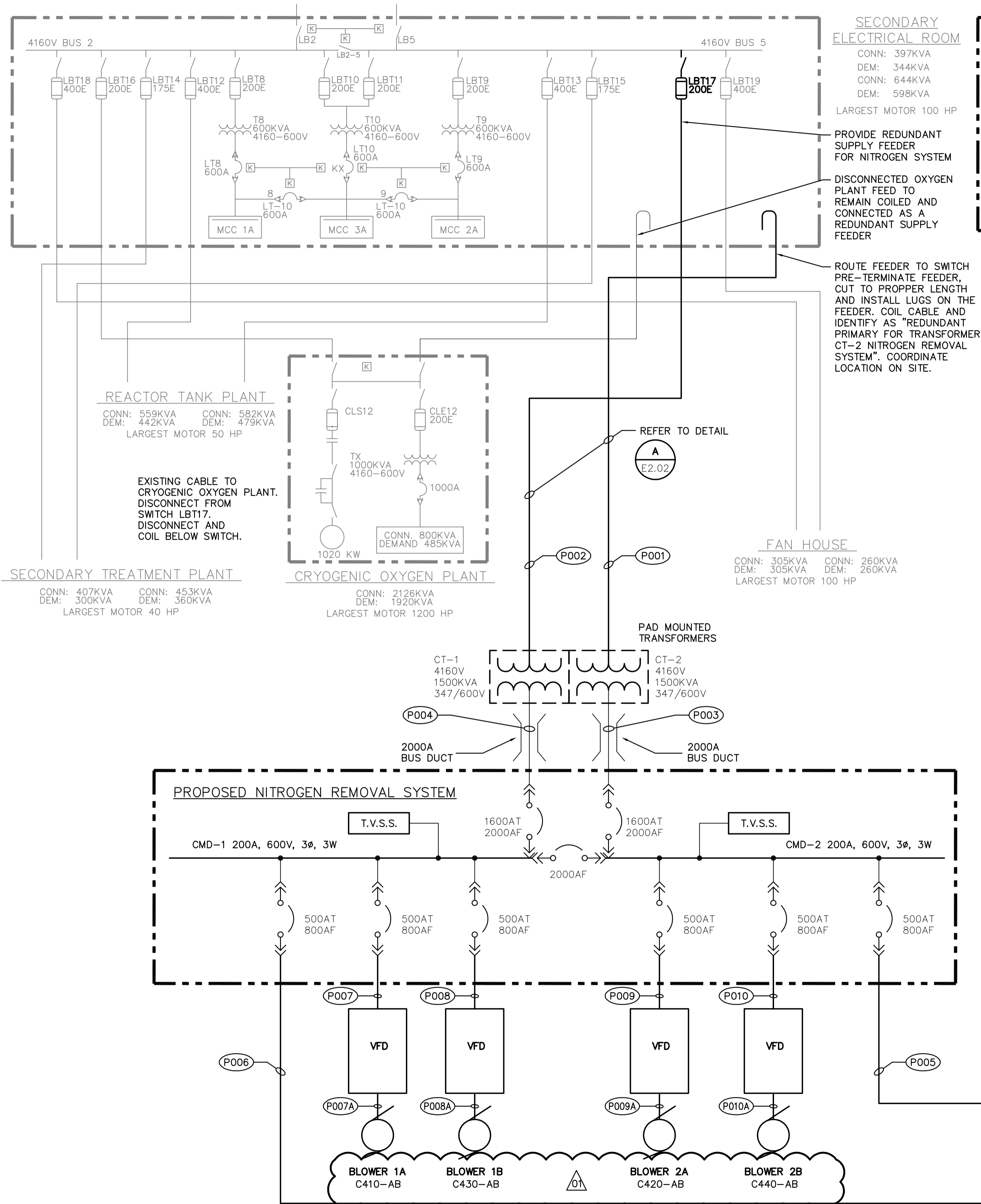
SINGLE LINE DIAGRAM SCALE: N.T.S.
