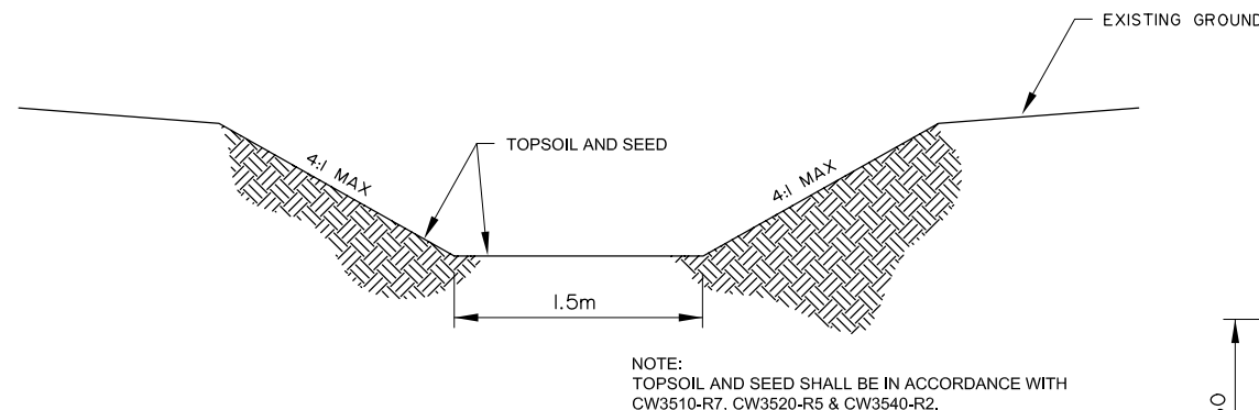
DITCH CROSS-SECTION N.T.S.
