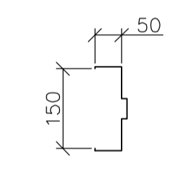
TYPE 1 FRAME TYPES SCALE: 1:10
