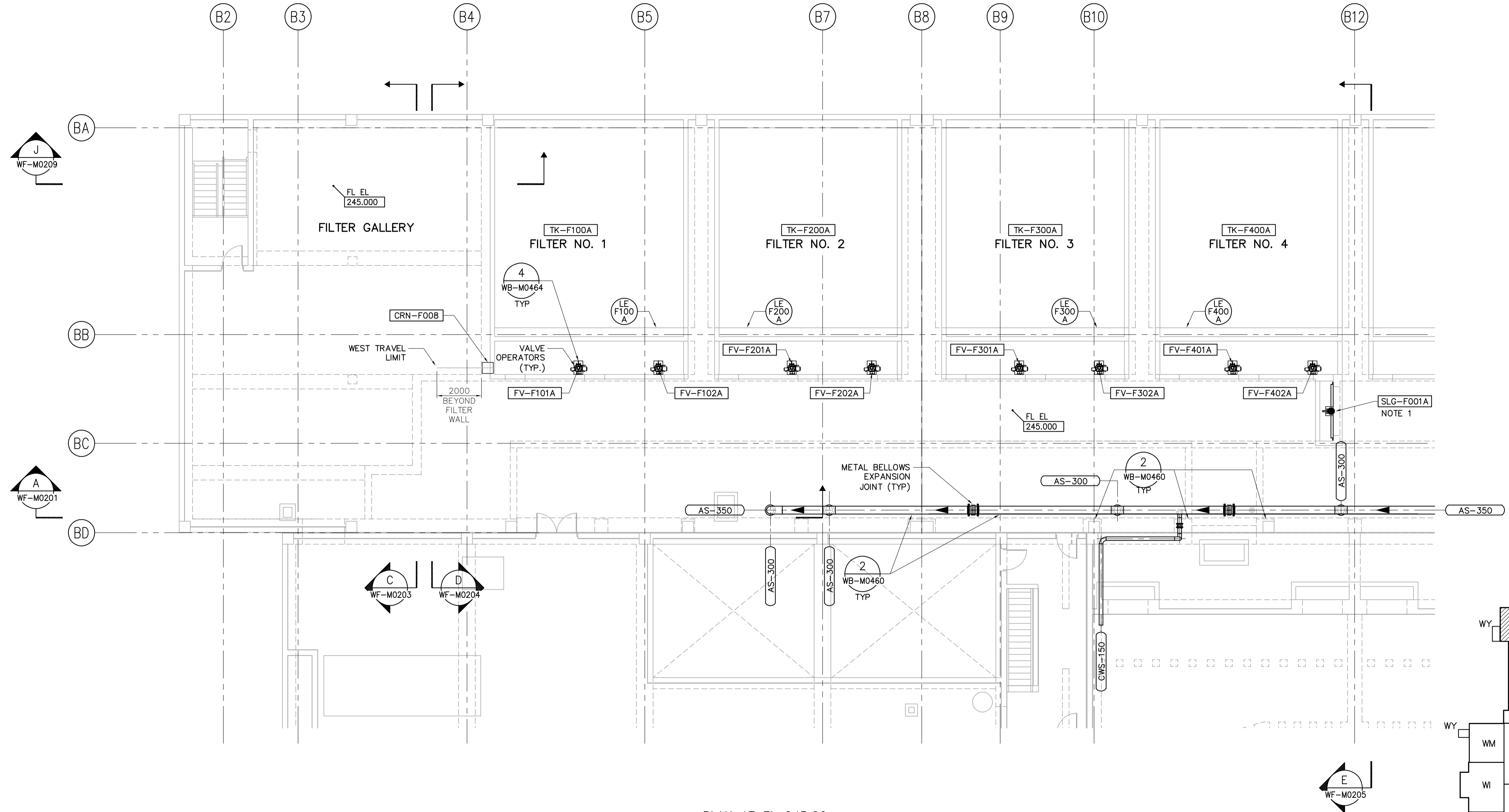
PLAN AT EL 245.00 1:100
