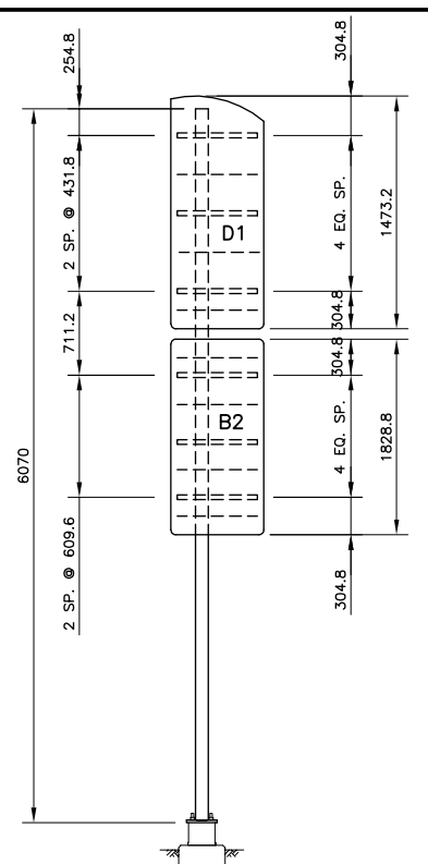
POST P6-R, SIGNS D1+B2
