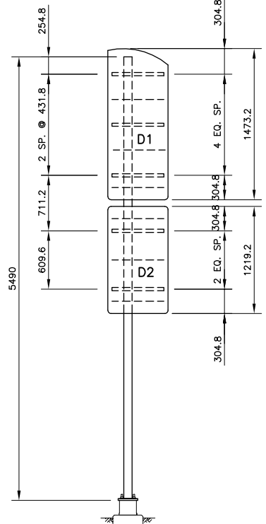
POST P10-R, SIGNS D1+D2
