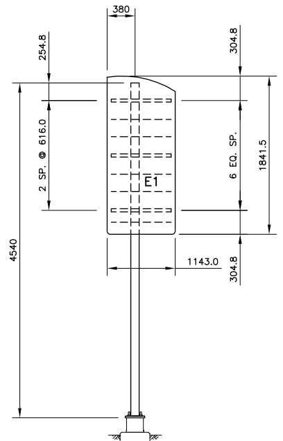
POST P11-R, SIGN E1
