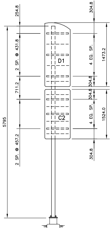
POST P9-R, SIGNS D1+C2
