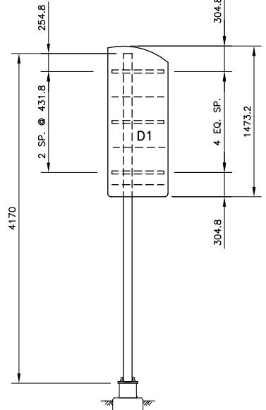
POST P4-R, SIGN D1
