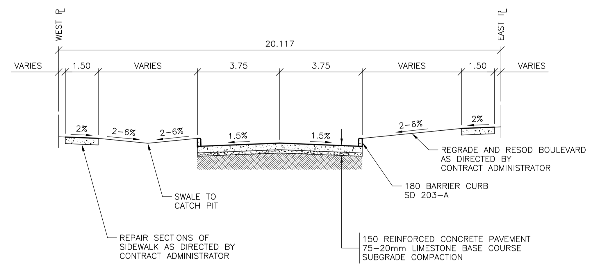
1 -- TYPICAL PAVEMENT CROSS SECTION 1 : 100 H, 1 : 50 V
