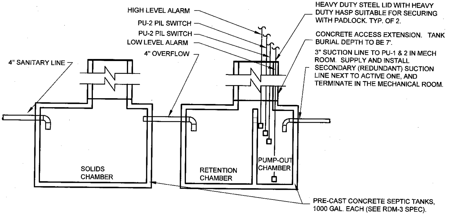
1 SEPTIC TANK DETAIL RDM2 SCALE: N.T.S.
