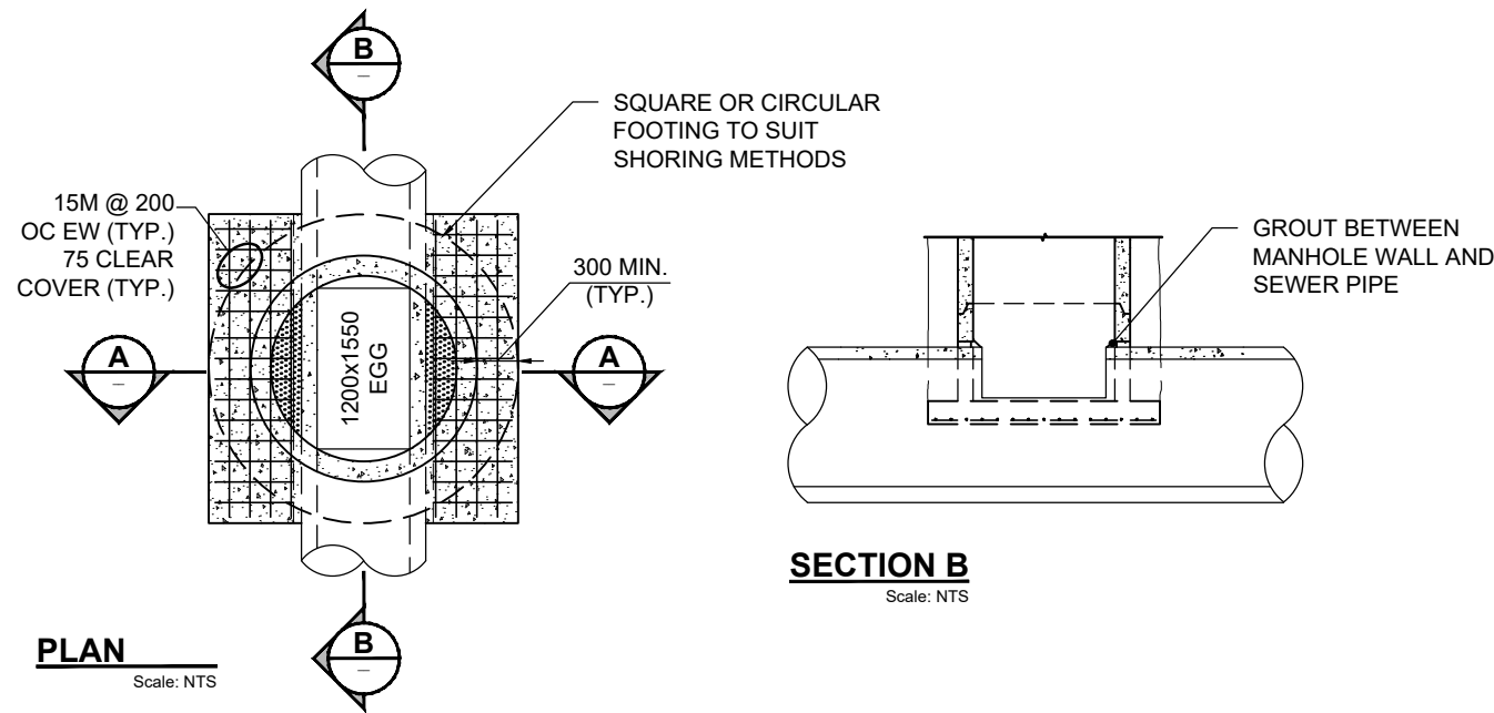
1 FULL MANHOLE REPLACEMENT DETAIL Scale: N.T.S.
