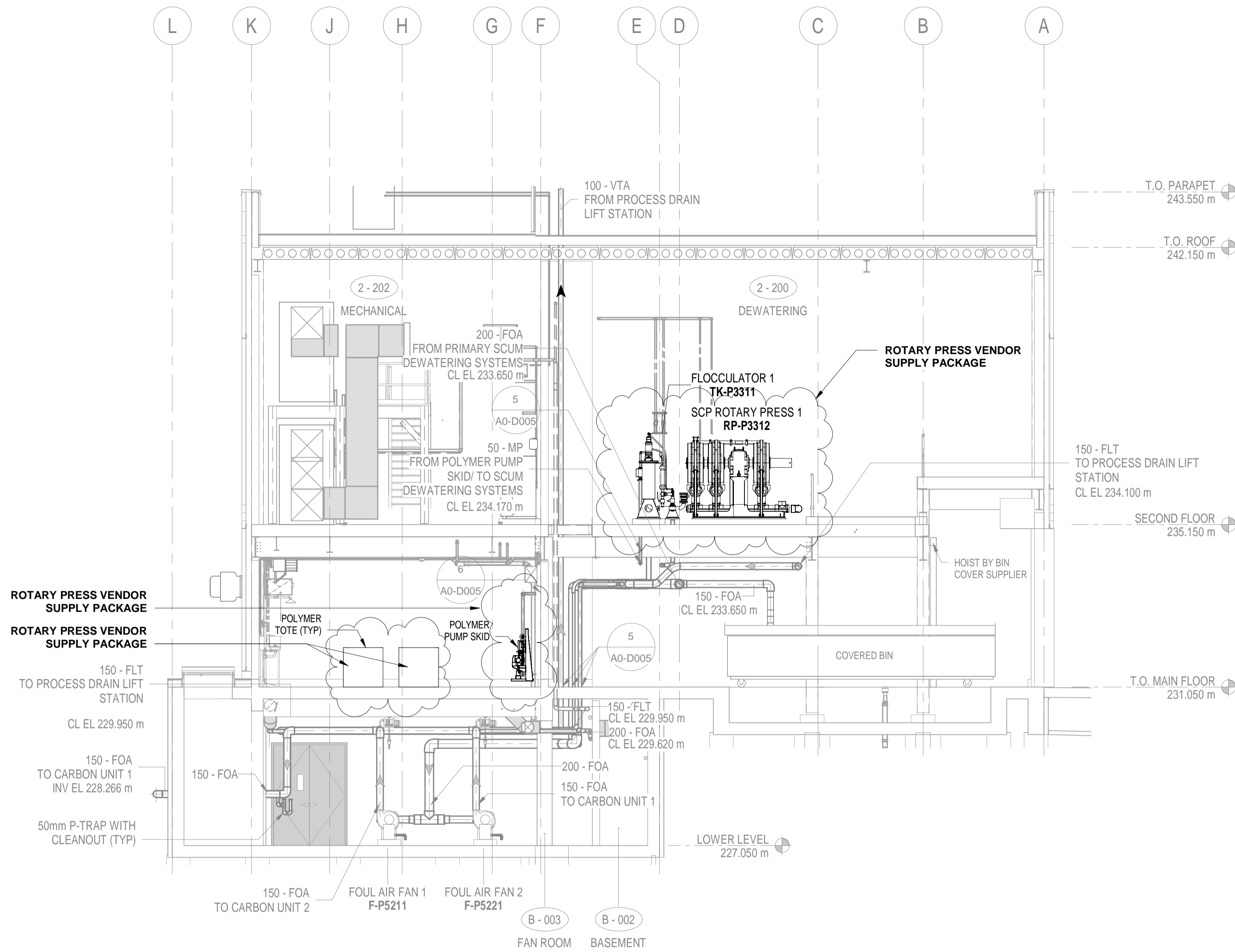
A SECTION P3-D101 SCALE: 1:75
