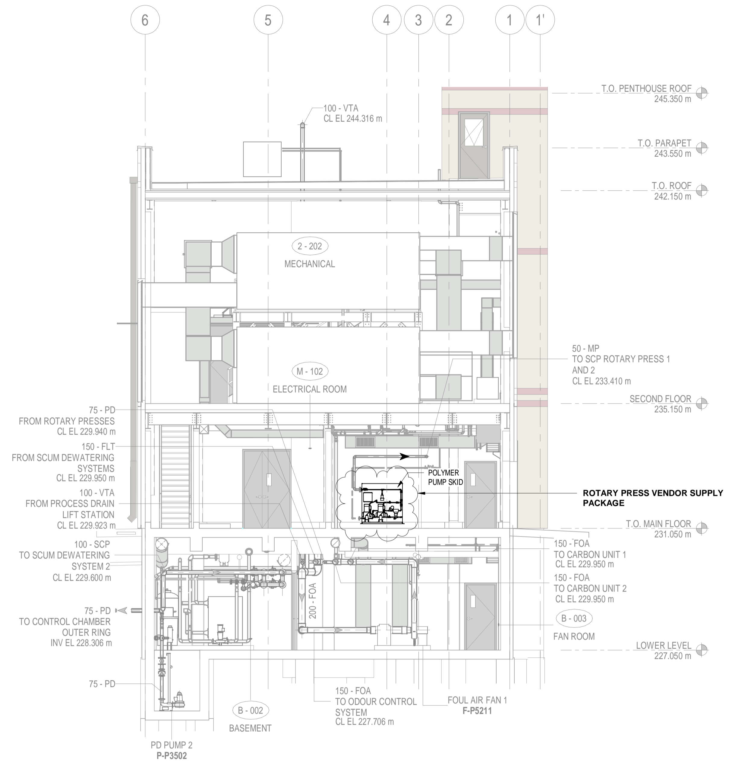
B SECTION P3-D101 SCALE: 1:75
