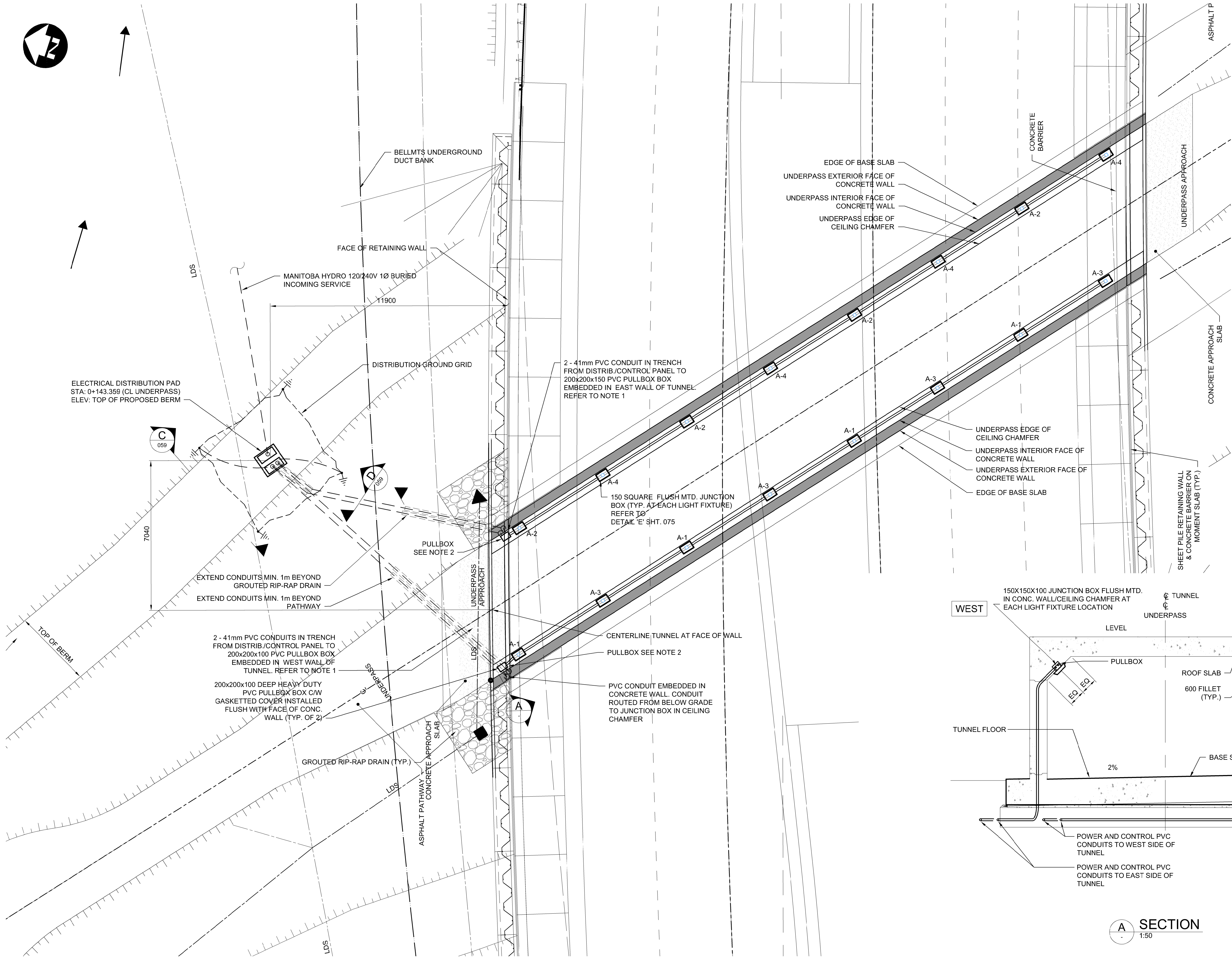
PLAN 1:100
