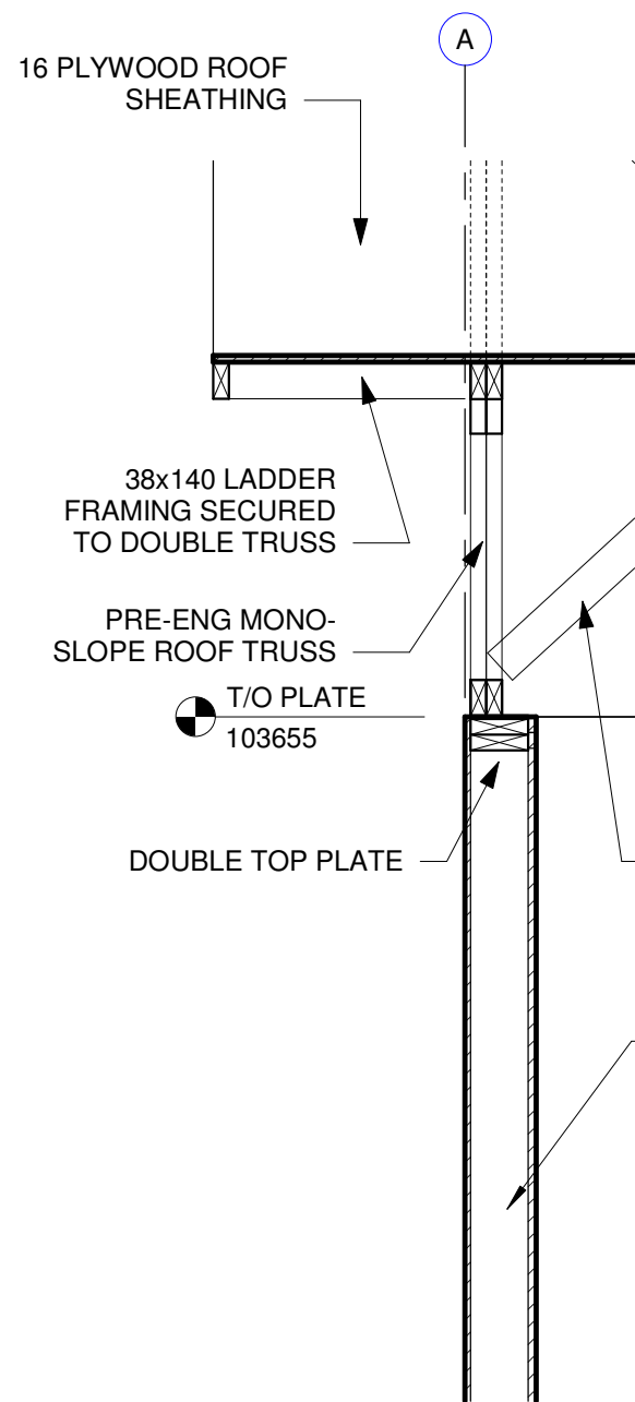
1 SECTION S502 1 : 20
