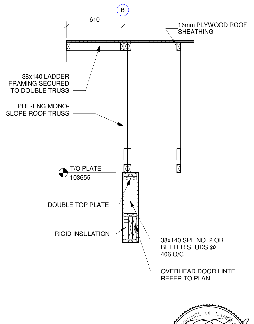
3 SECTION S502 1 : 20
