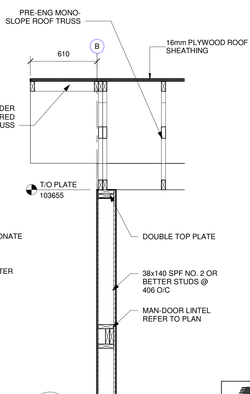
2 SECTION S502 1 : 20
