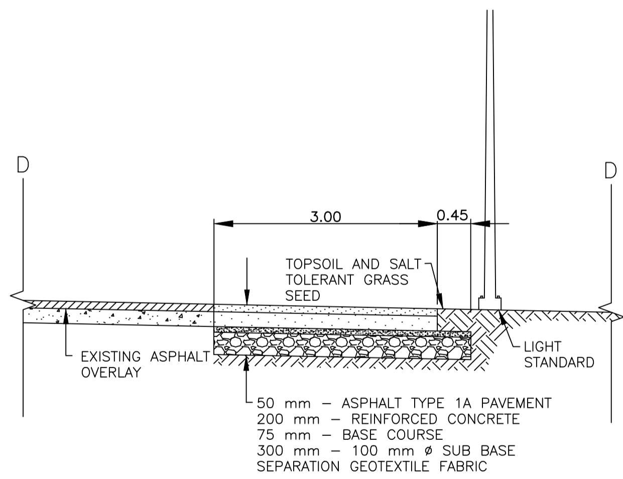
CROSS SECTION D-D N.T.S.
