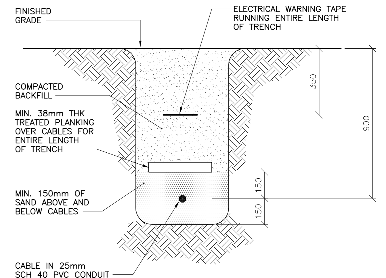
3 TRENCH DETAIL N.T.S.
