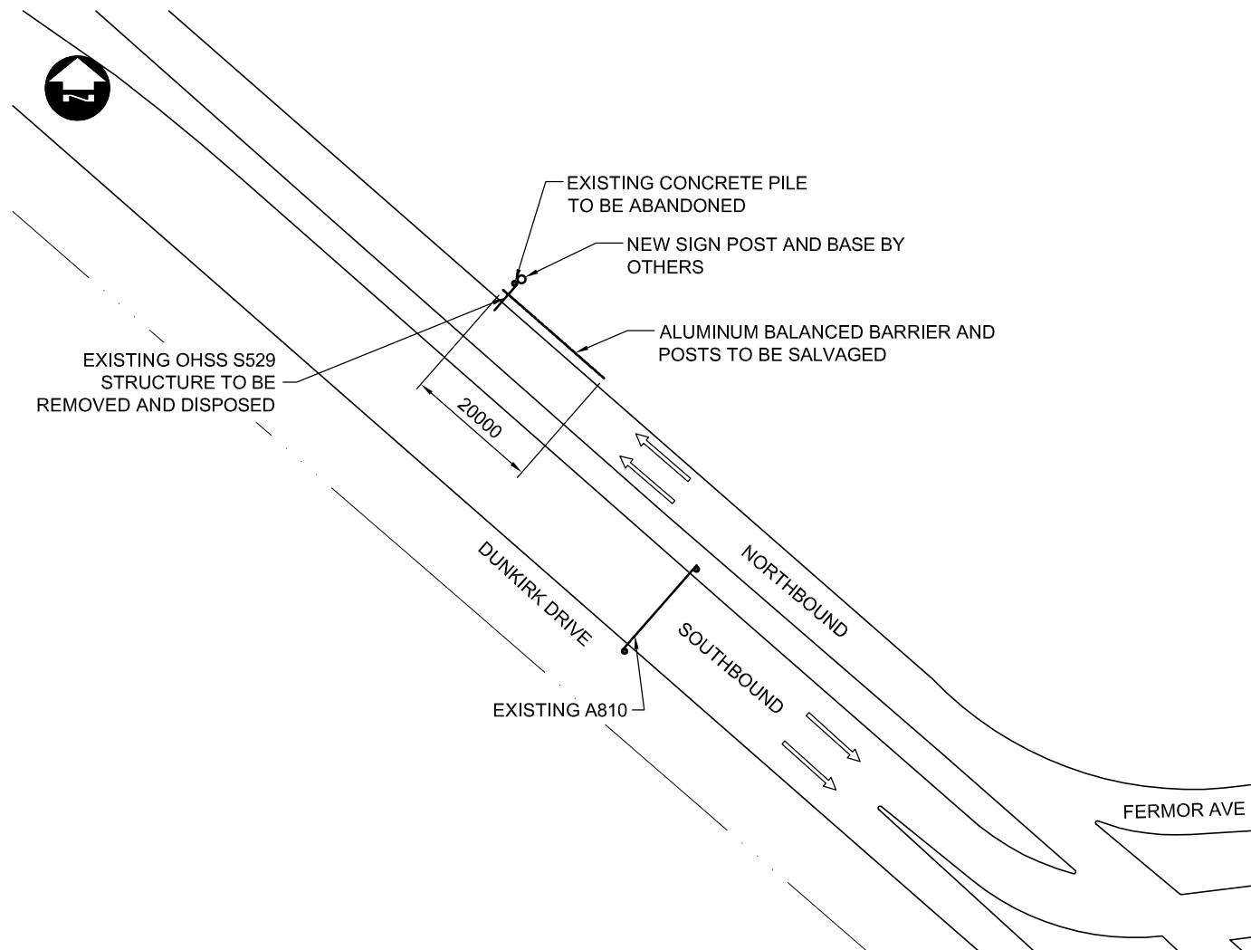
SITE PLAN 1:1,000
