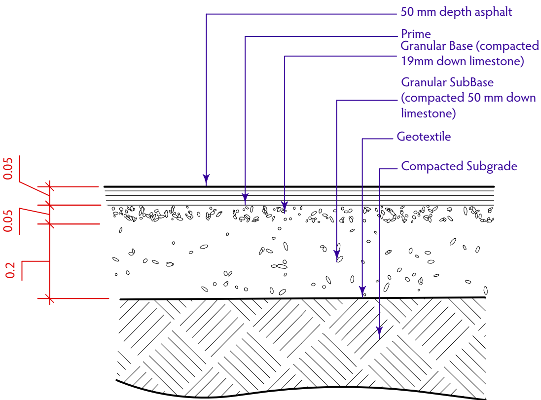
3 Light Duty Asphalt L-10 Scale: 1:10
