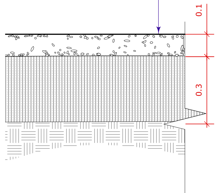
4 Local Wood Chip Mulch Planting Bed L-10 Scale: 1:10
