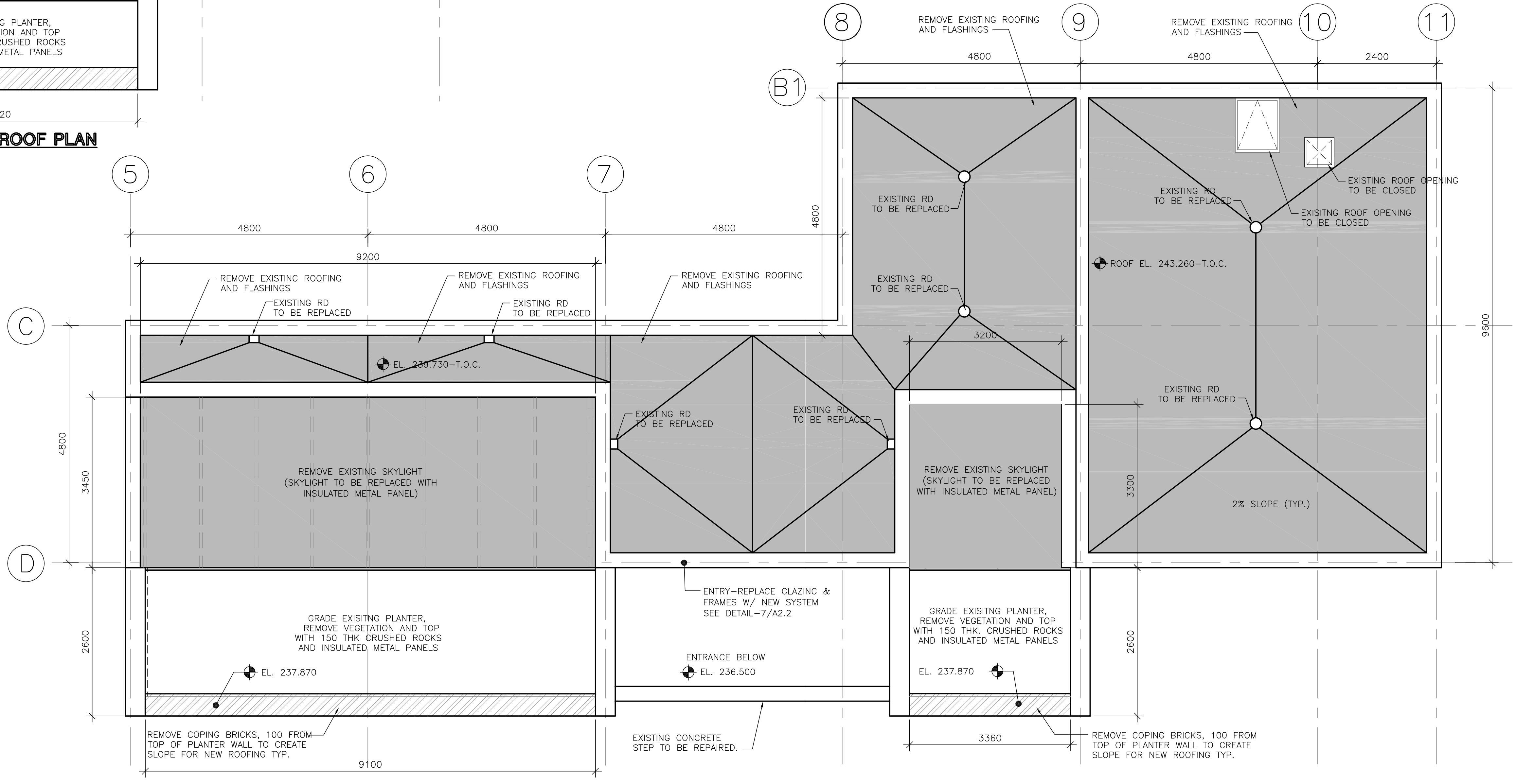
1 EXISTING ROOF PLAN A1.1 SCALE: 1:50
