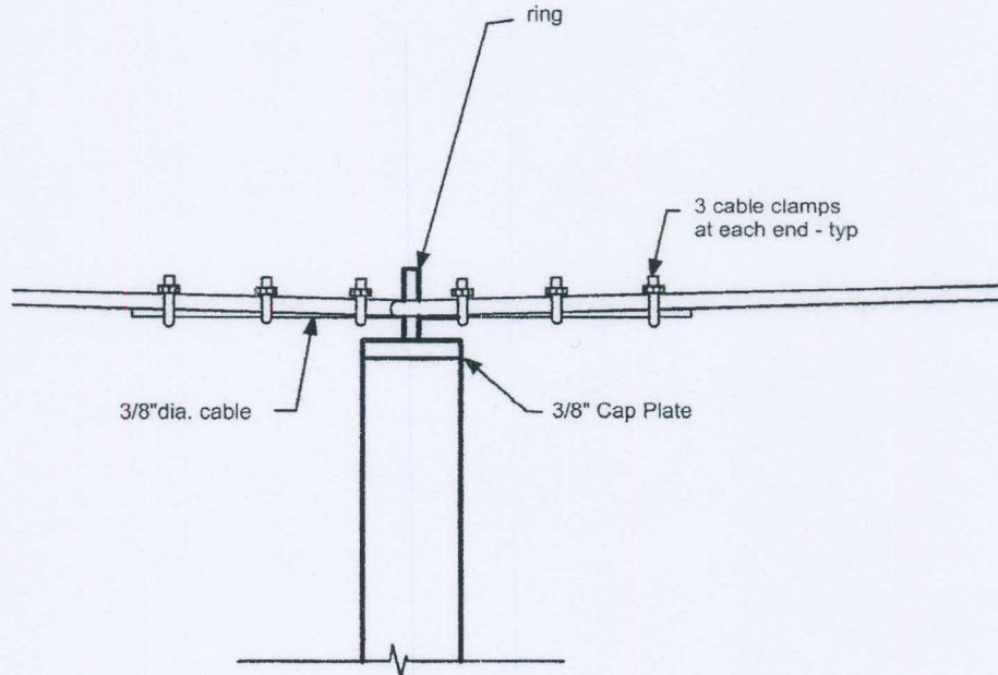
1 SECTION DETAIL S-0 SCALE: 3/4" = 1'-0"
