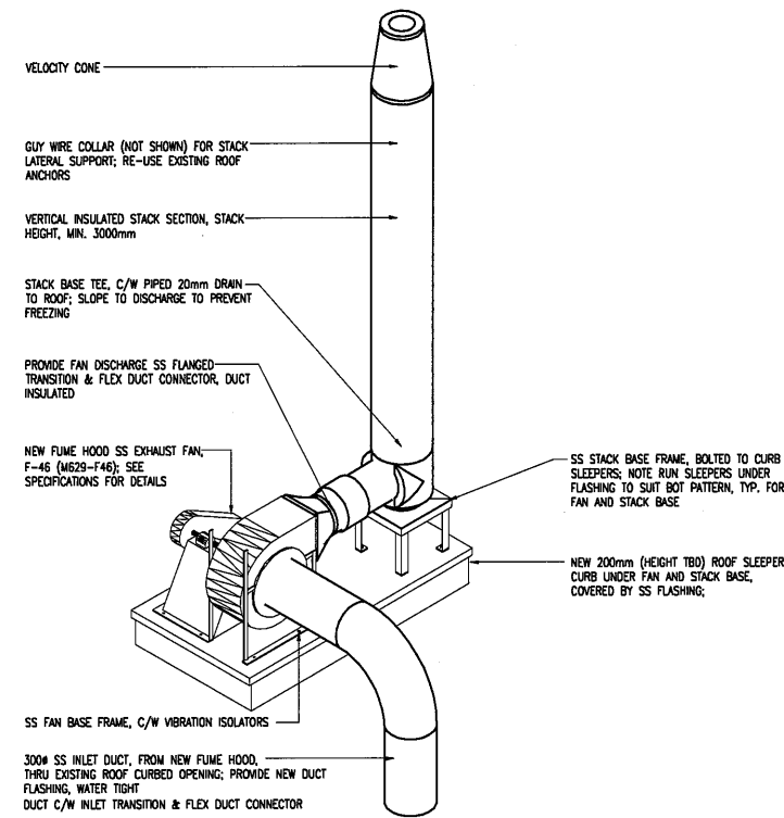
DETAIL - EXHAUST FAN F-46 SCALE NTS
