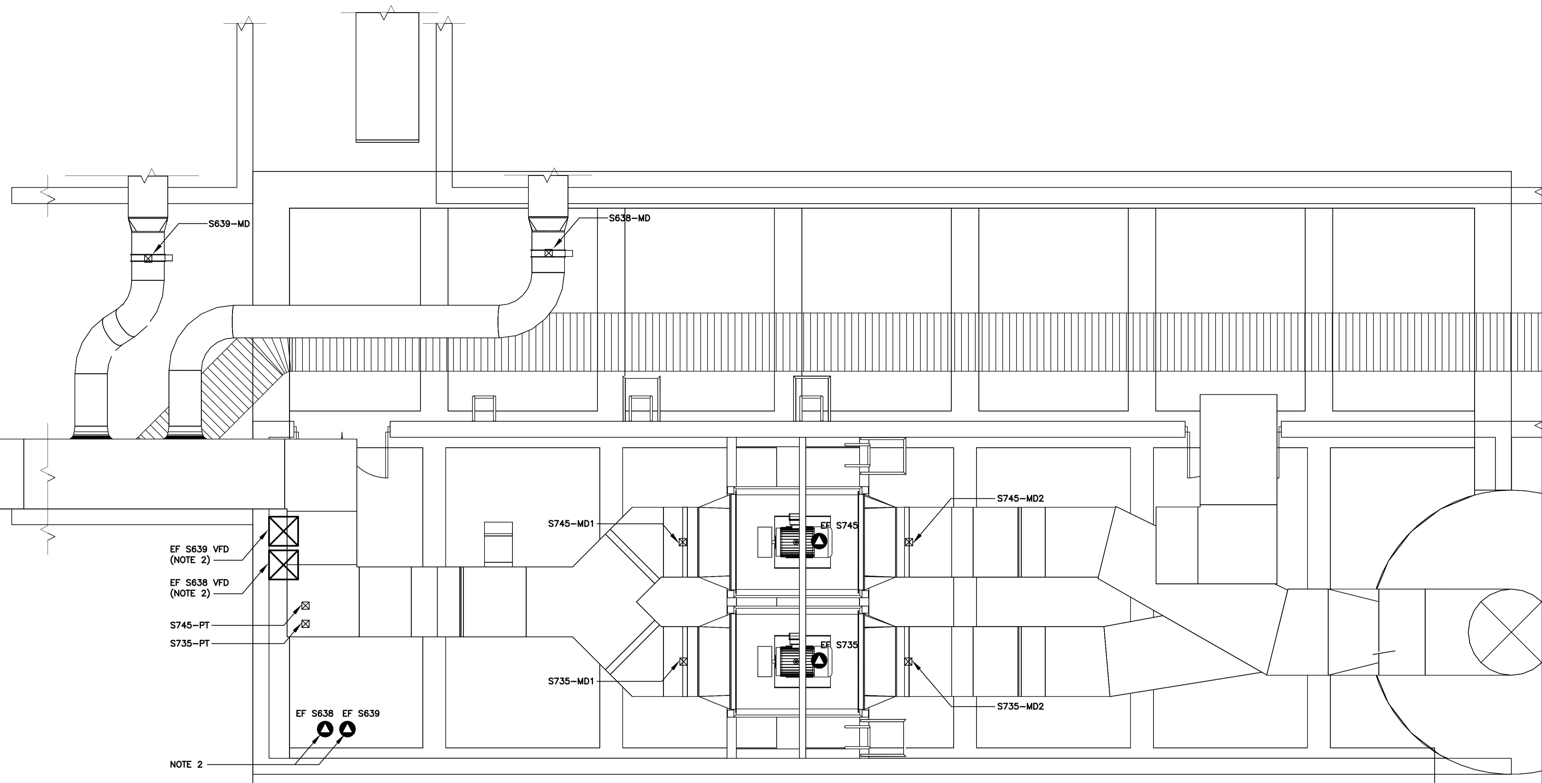
A ODOUR DISPERSION ROOM - PLAN SCALE: 1:50
