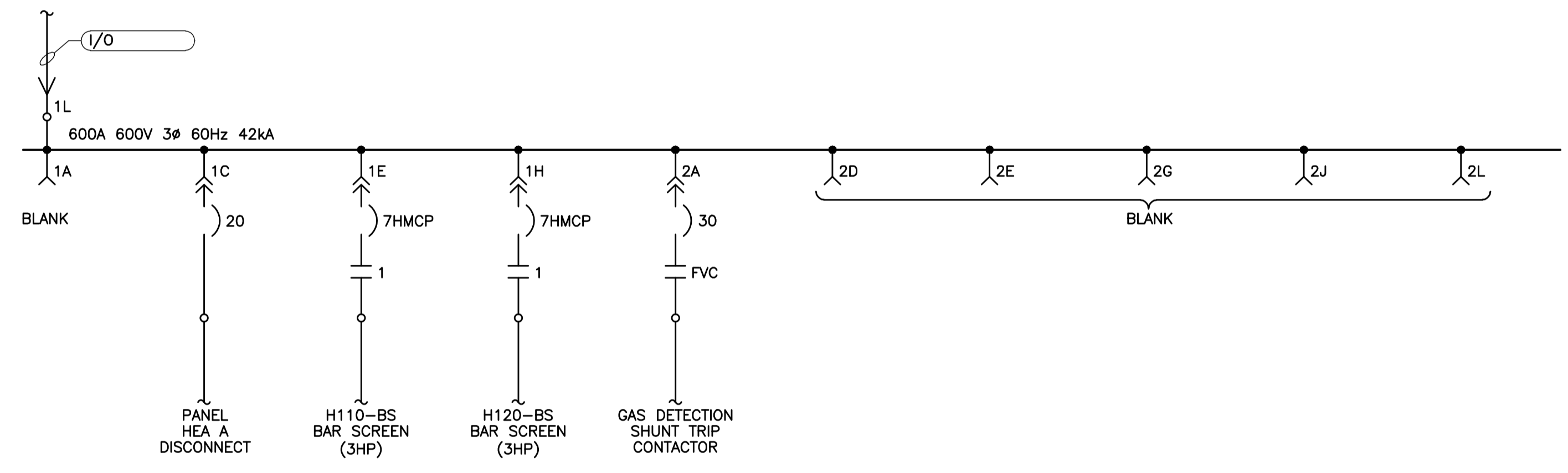
2 MCC-HE SINGLE LINE DIAGRAM SCALE: N.T.S.
