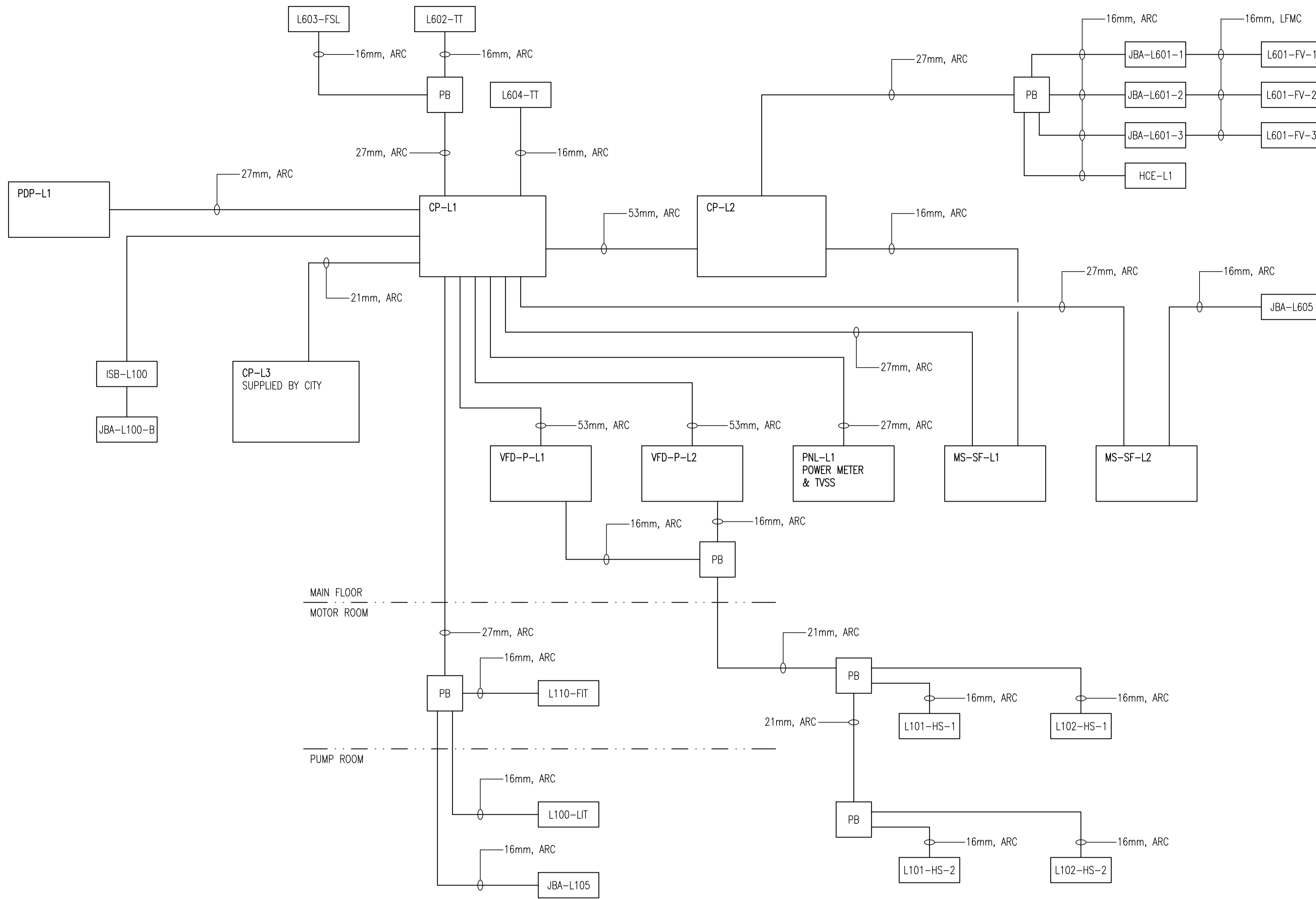
AUTOMATION CONDUIT RISER DIAGRAM SCALE: NTS
