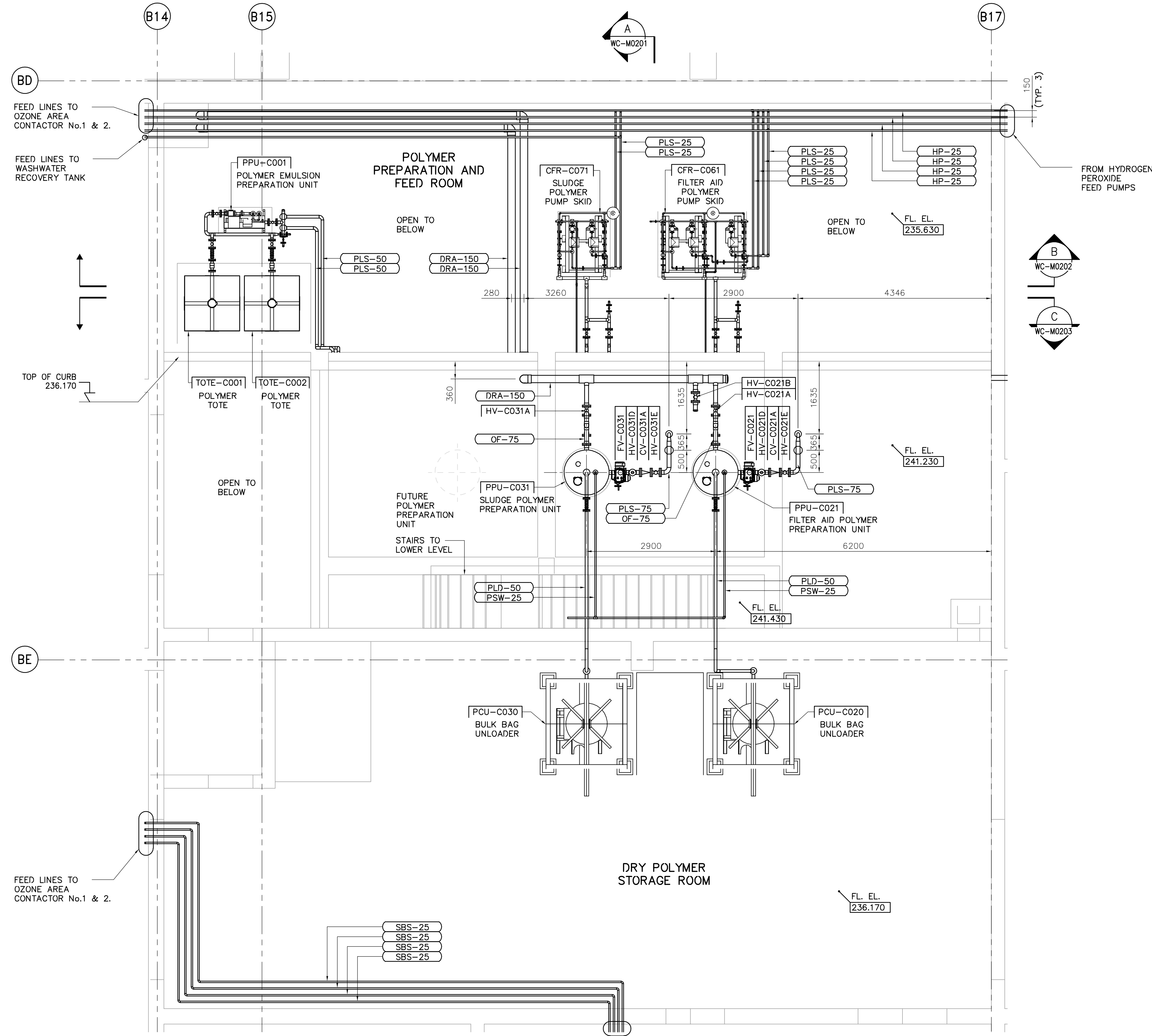
1 WC-M0121 1:50 DETAIL
